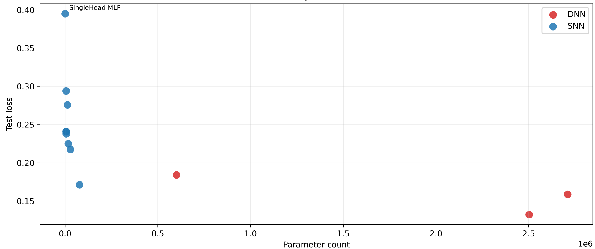
Test loss vs parameter count
