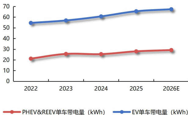
图表 2：新能源车单车带电量逐步提升
