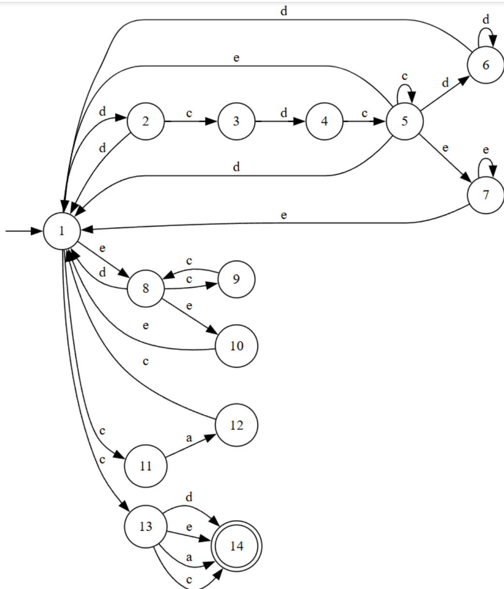
Рис. 2: Диаграмма НКА
