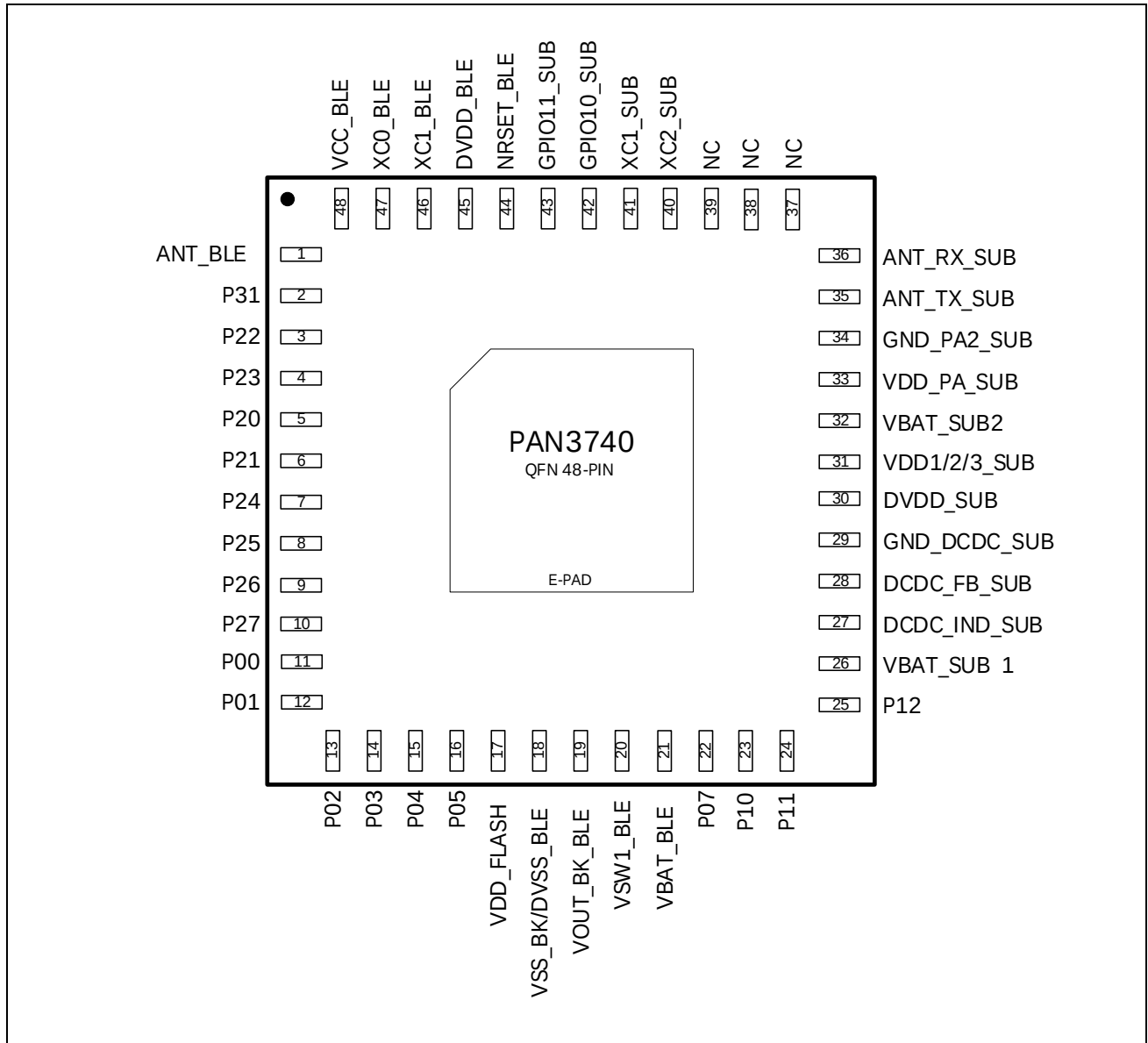
图 4-1 QFN48 引脚图
