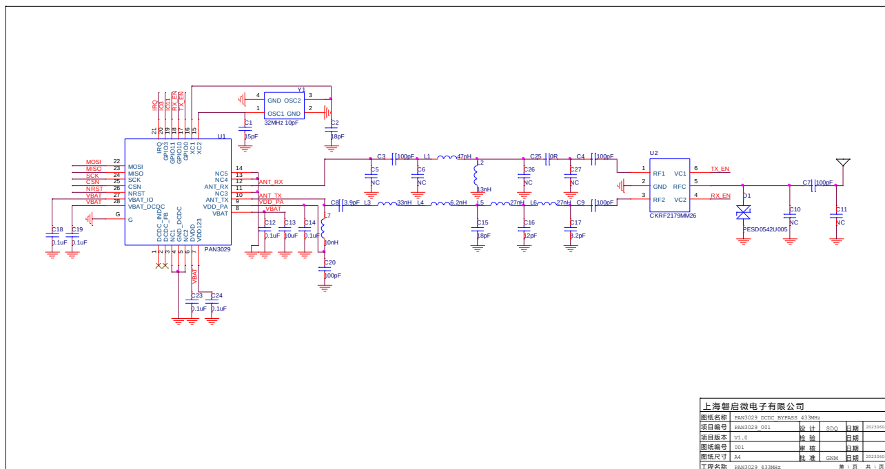
图 13-1 LDO Mode 433MHz 参考原理图
