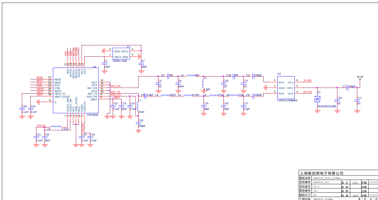
图 13-2 DCDC Mode 433MHz 参考原理图
