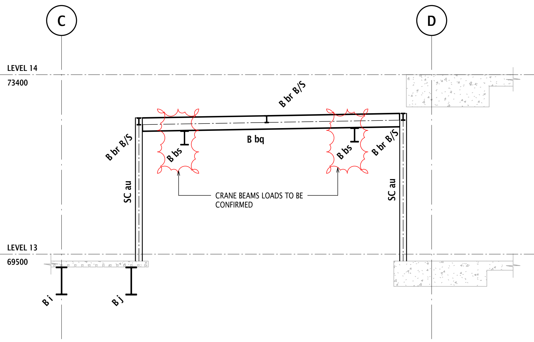
SECTION C SCALE 1 : 50
