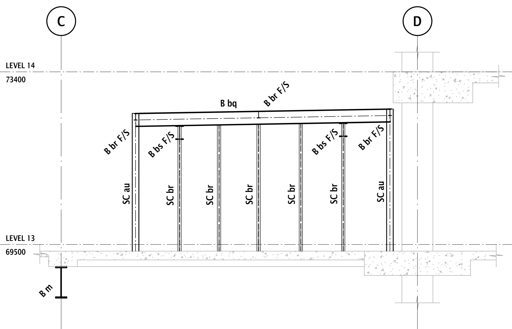
SECTION B SCALE 1 : 50
