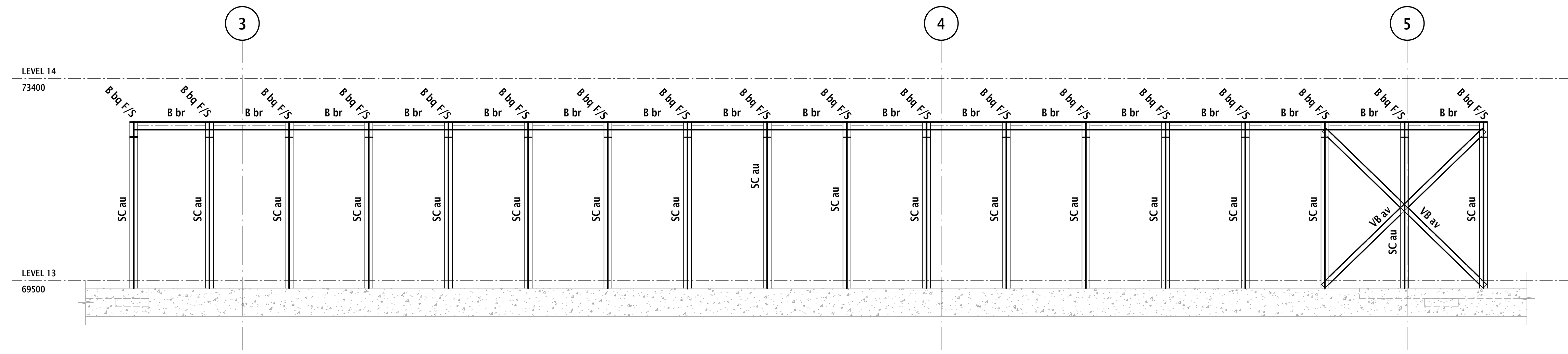
SECTION A SCALE 1 : 50
