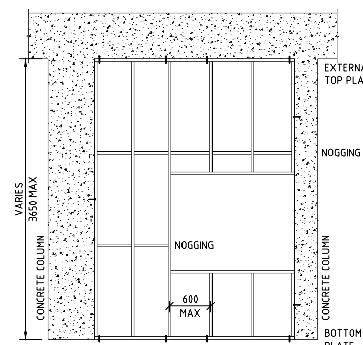
92mm WIDE STUD FRAMING N.T.S.
