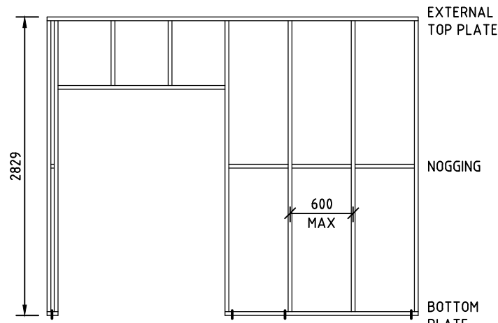
76mm WIDE STUD FRAMING N.T.S.
