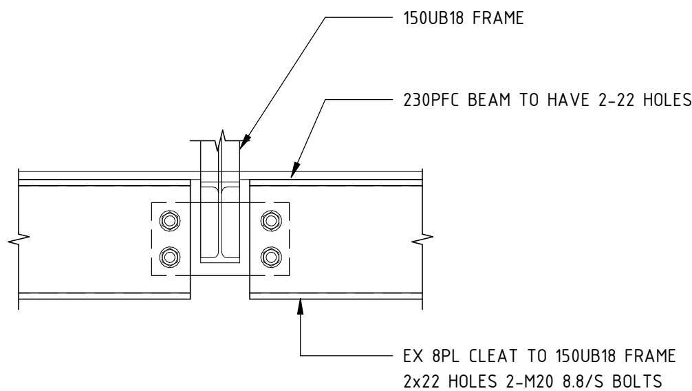
SECTION 3 1 : 10 12-A-152-ST0261
