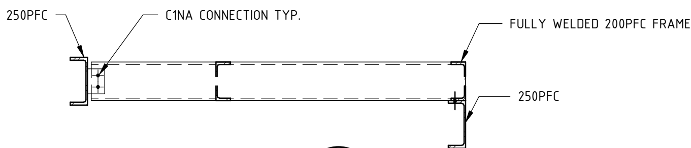
SECTION 6 1 : 20 12-A-152-ST0261
