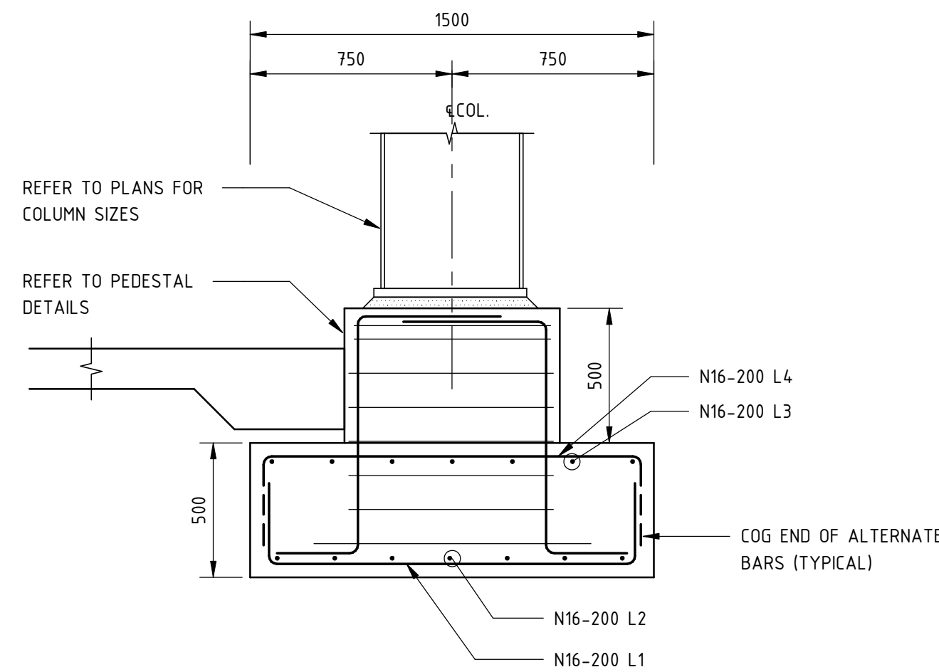
SECTION 4 1 : 20
