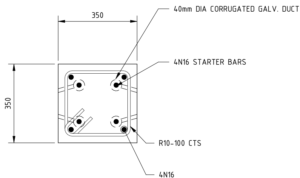
SECTION A-1 1 : 10
