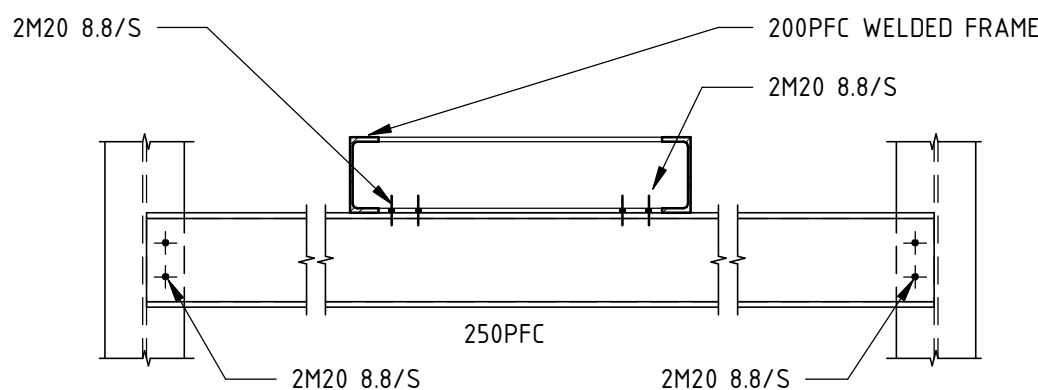
SECTION 7 1 : 20 12-A-152-ST0261
