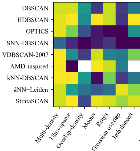
Target F1
