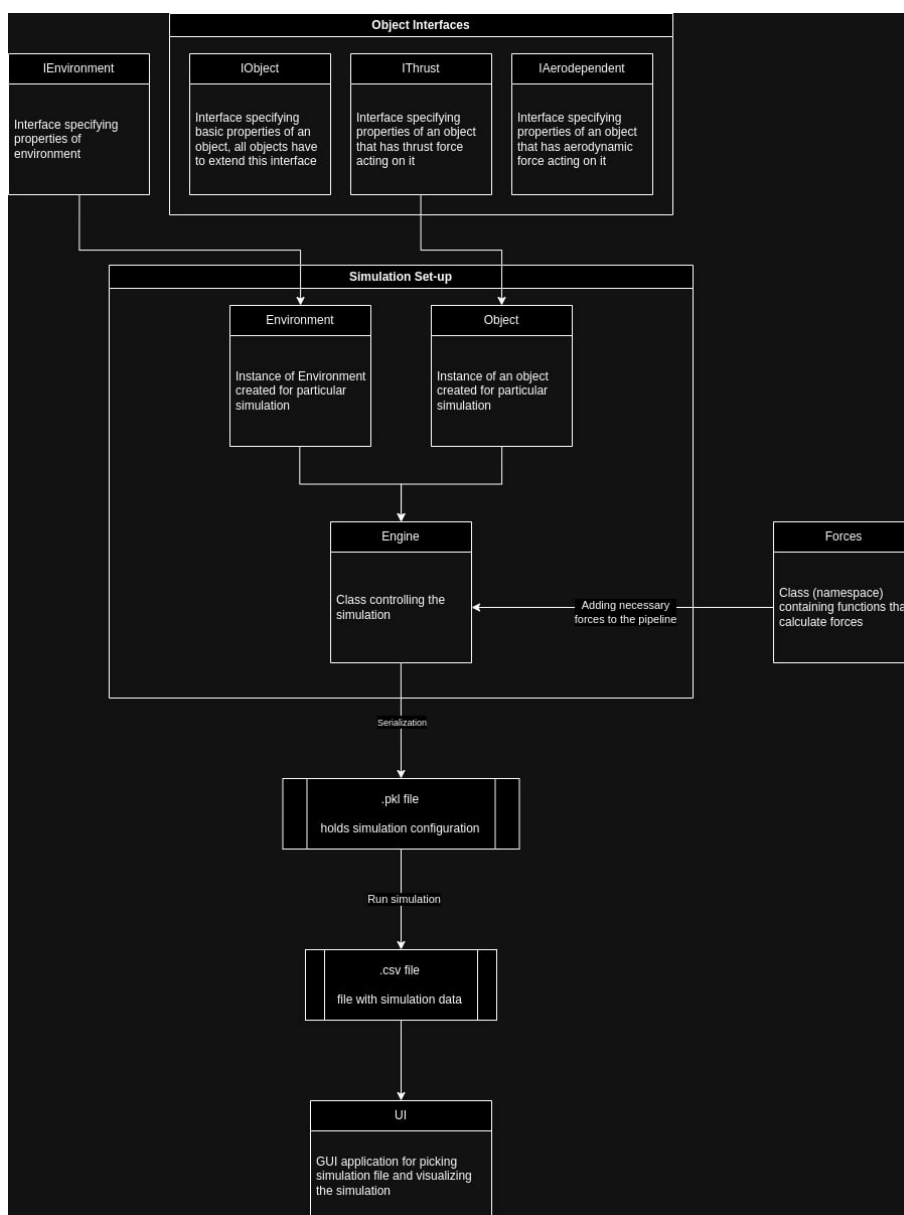
Rysunek 2.1. Architektura systemu symulacji, Źródło: Opracowanie własne.
