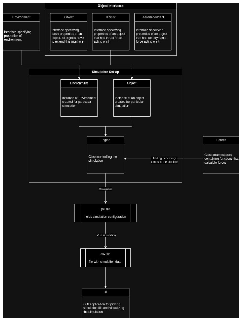
Rysunek 2.9. Architektura systemu symulacji, Źródło: Opracowanie własne.
