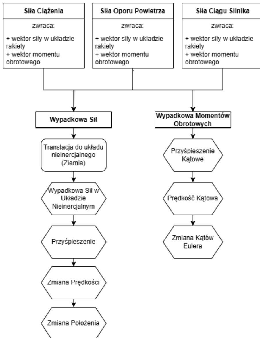
Rysunek 2.10. Schemat działania sił w symulacji, Źródło: Opracowanie własne.
