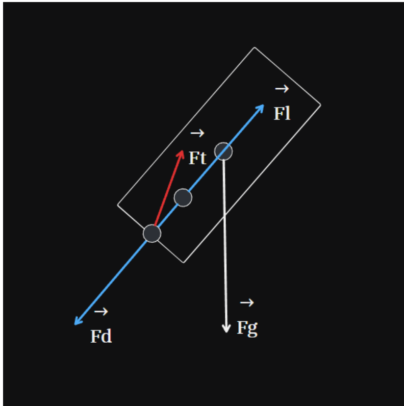
Rysunek 2.1. Siły działające na raketę w locie, źródło: Opracowanie własne.
