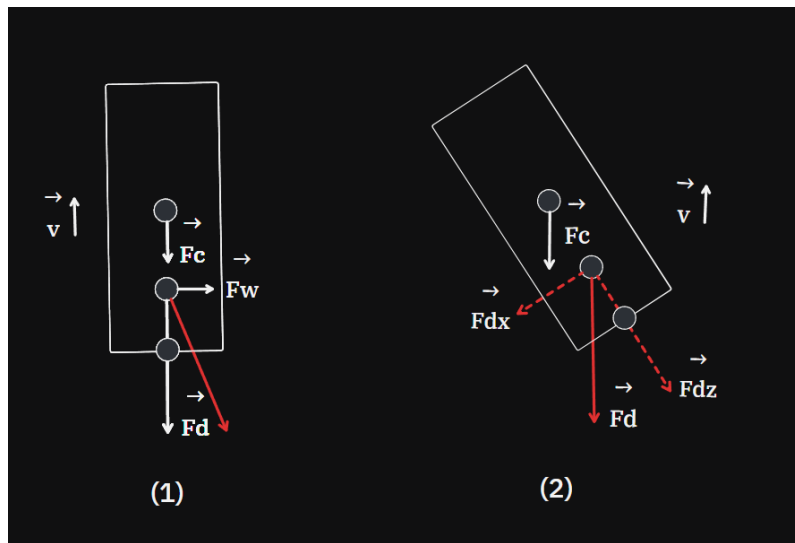
Rysunek 2.6. Przykład działania sił stabilizujących raketę w locie, źródło: Opracowanie własne.
