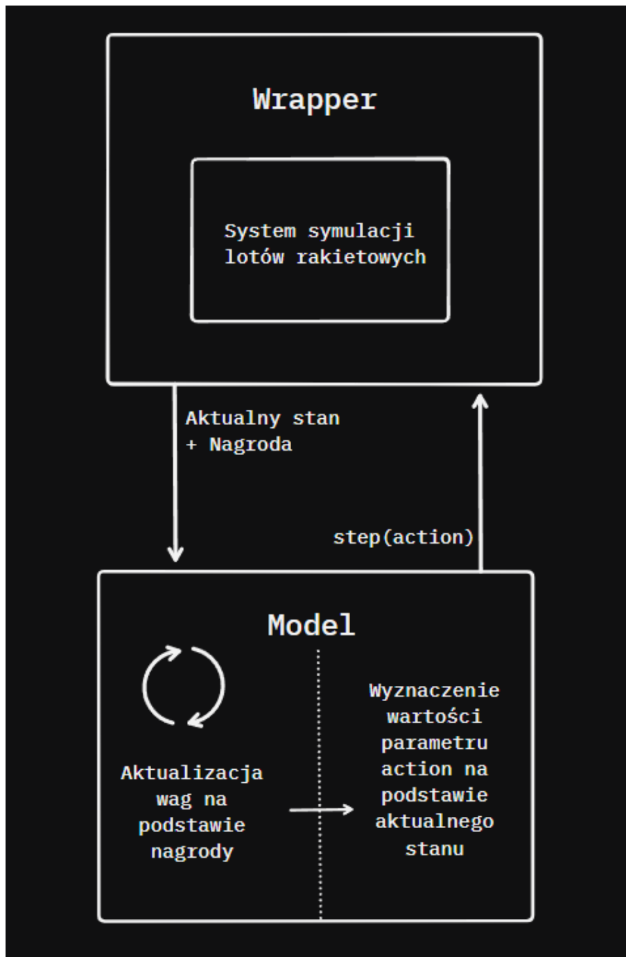
Rysunek 3.1. Schemat architektury systemu uczącego. Opracowanie własne.
