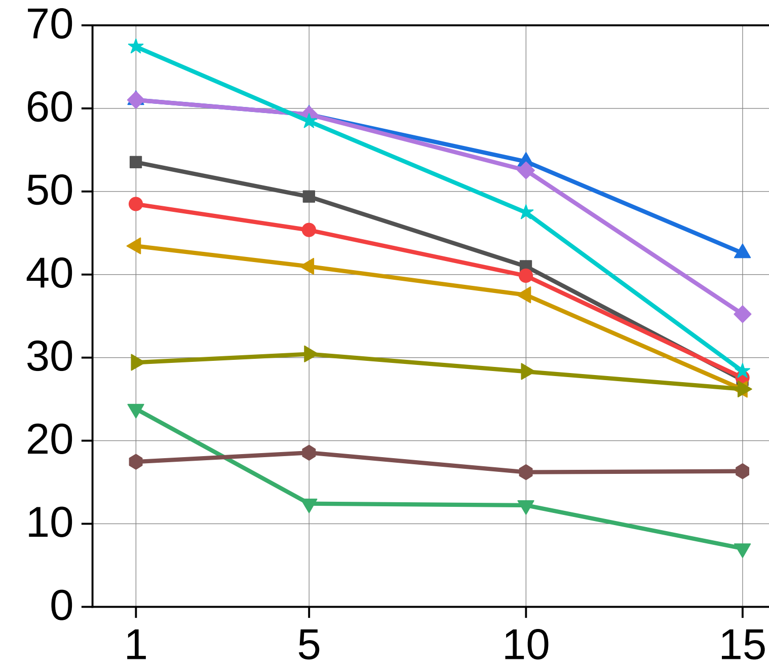
(b) Devign
