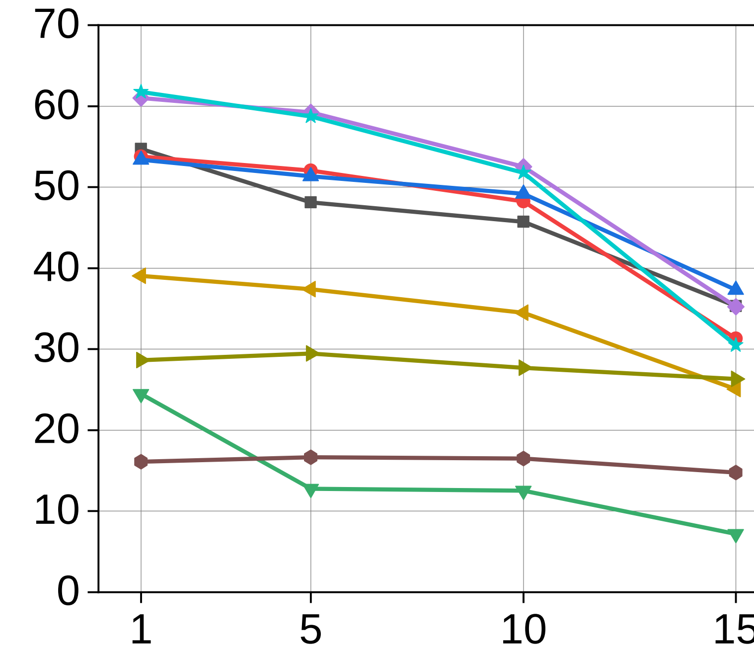
(d) Reveal
