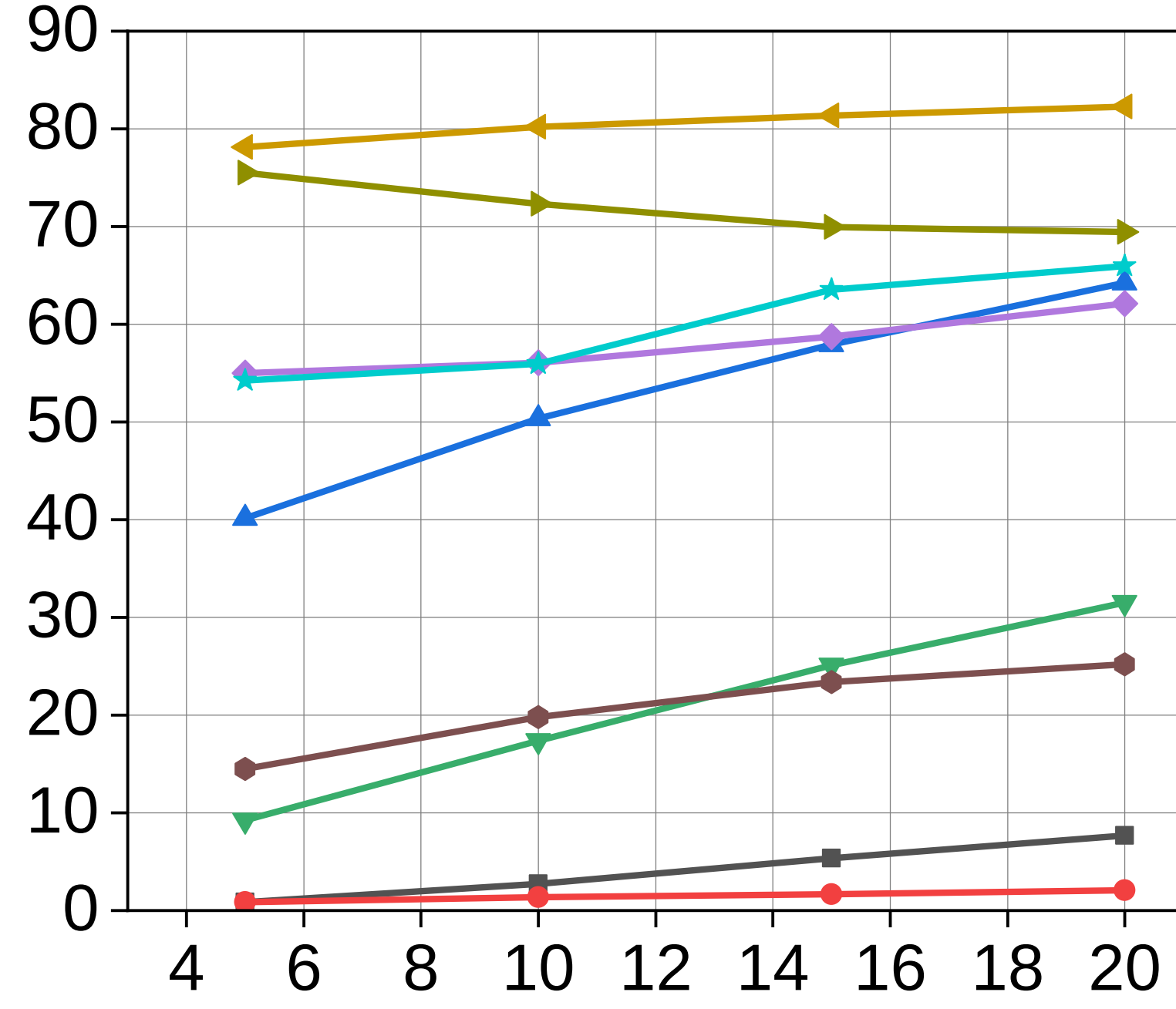
(d) Reveal
