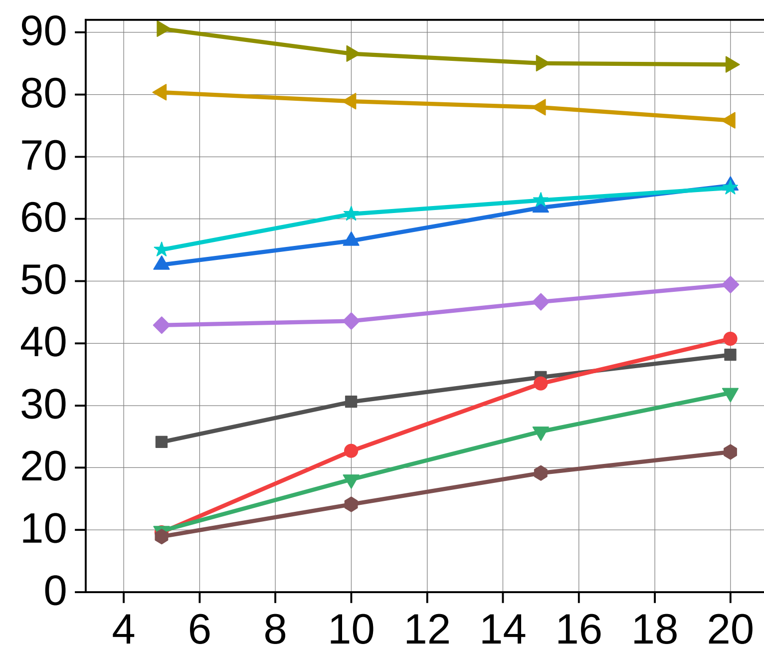
(b) Devign
