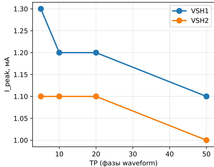
Пиковый ток (95-й перцентиль)
