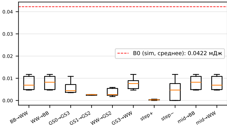
Распределение энергии по точкам Парето-фронта (10 сценариев)
