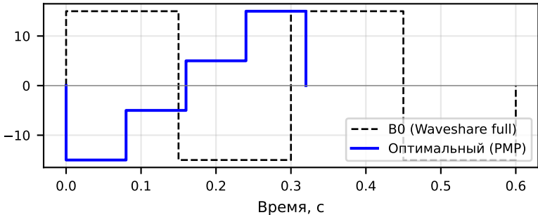
Найденный waveform vs заводская LUT (переход GS0→GS3)
