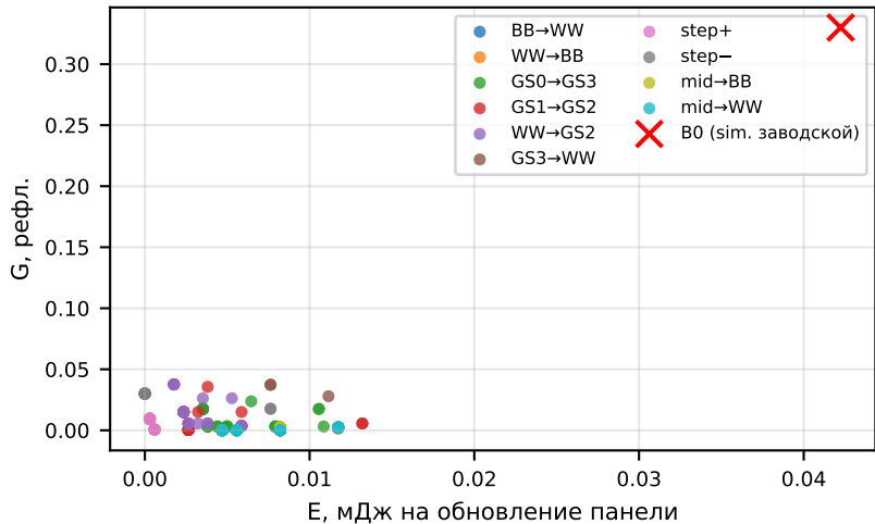
Парето-фронт (проекция E,G) на 10 сценариях
