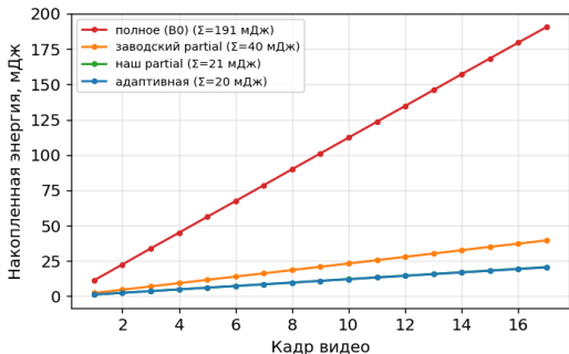
Накопленная энергия за сцену (множество Жюлиа, 17 кадров)
