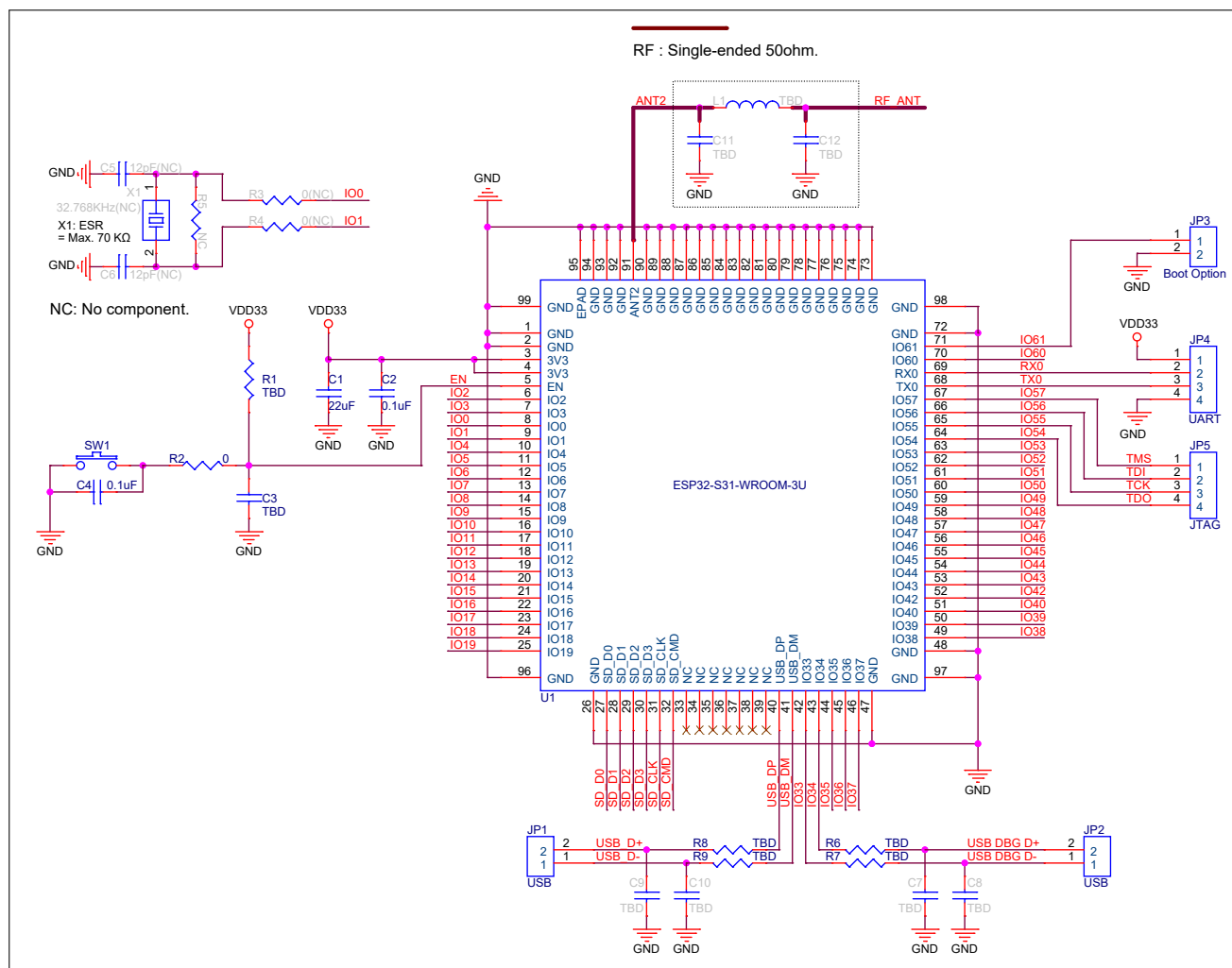
图 9-2. ESP32-S31-WROOM-3U 外围设计原理图
