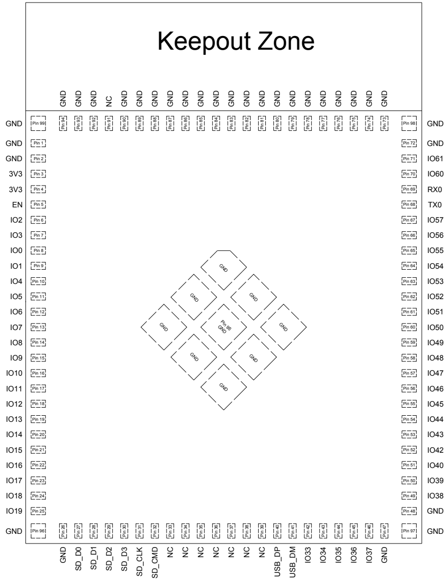
图 3-1. ESP32-S31-WROOM-3 管脚布局（顶视图）
