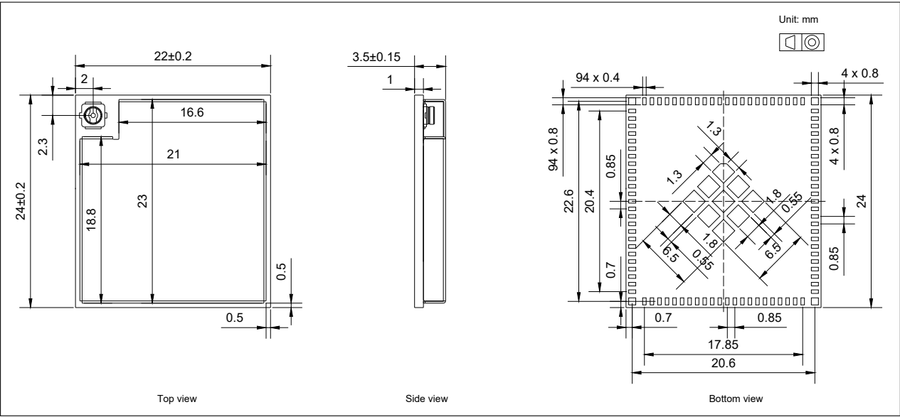
图 10-2. ESP32-S31-WROOM-3U 模组尺寸
