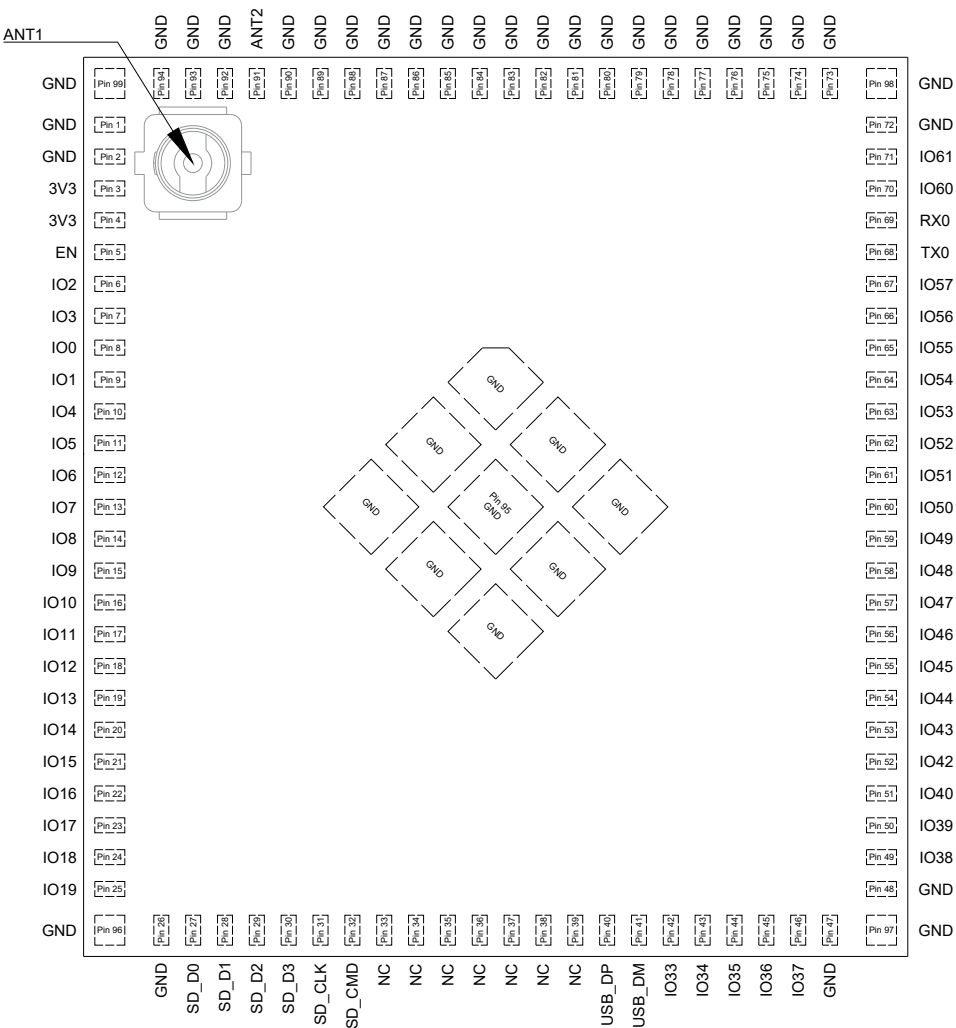
图 3-2. ESP32-S31-WROOM-3U 管脚布局（顶视图）
