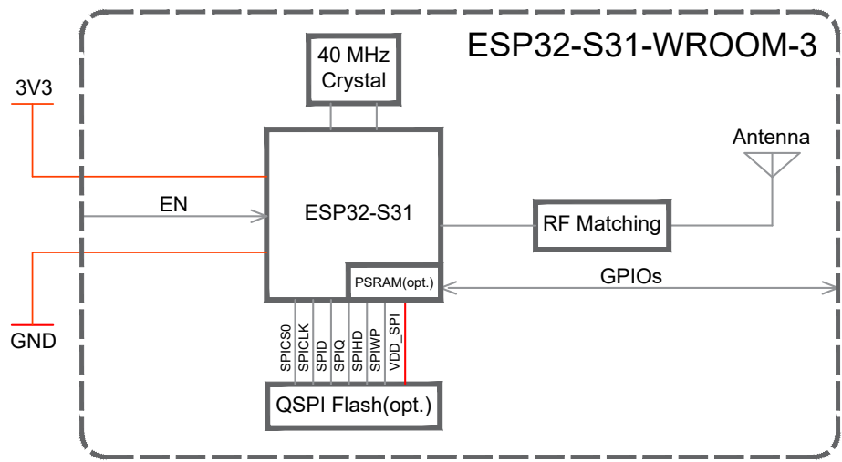
图 2-1. ESP32-S31-WROOM-3 功能框图
