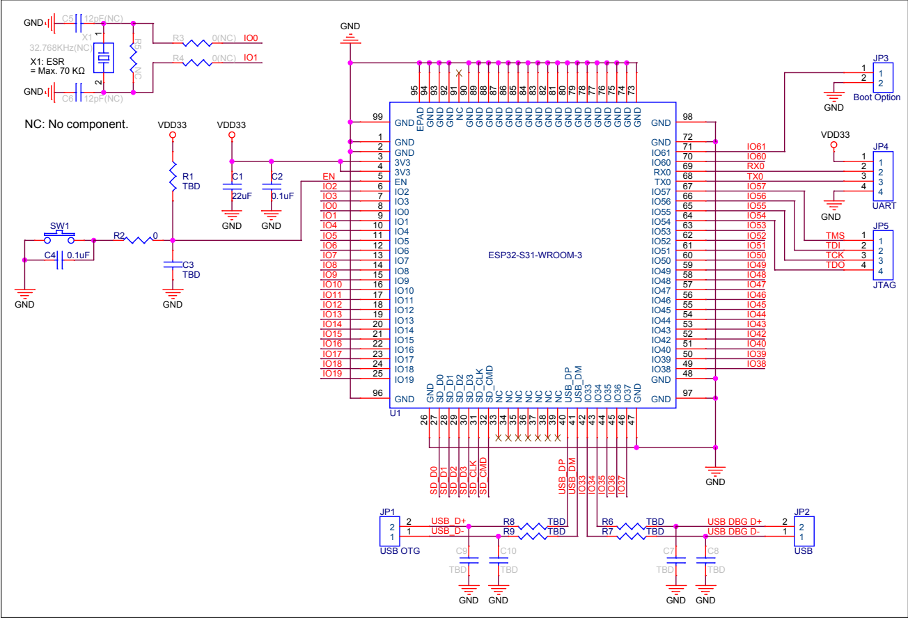
图 9-1. ESP32-S31-WROOM-3 外围设计原理图
