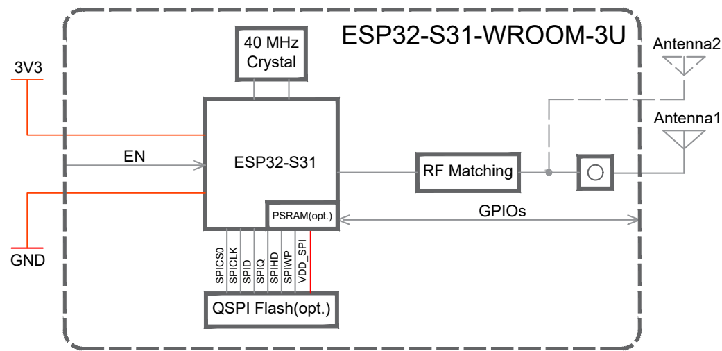
图 2-2. ESP32-S31-WROOM-3U 功能框图
