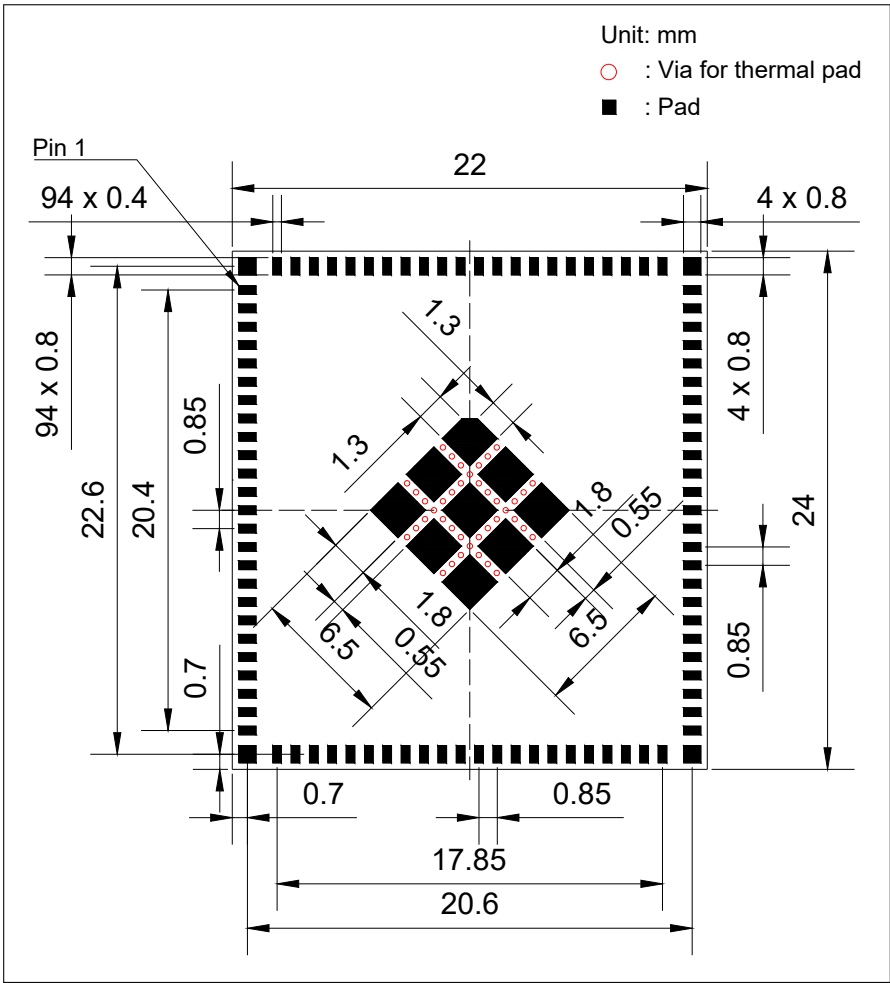
图 11-2. ESP32-S31-WROOM-3U 推荐 PCB 封装图形
