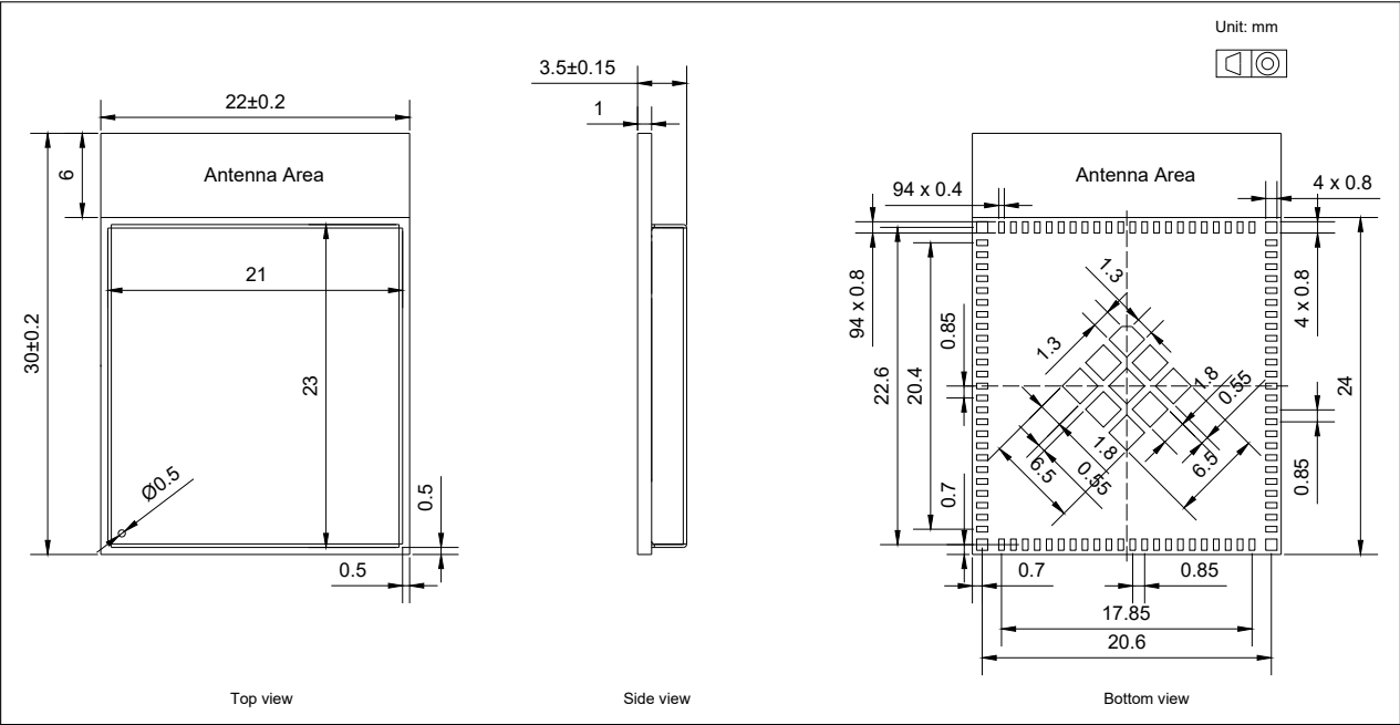
图 10-1. ESP32-S31-WROOM-3 模组尺寸
