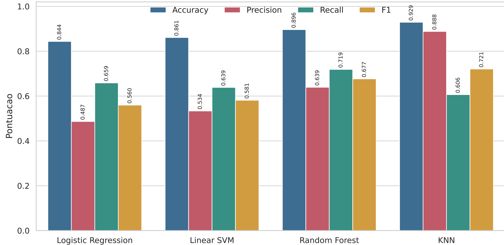
Desempenho dos baselines leves na deteccao de mutantes equivalentes
