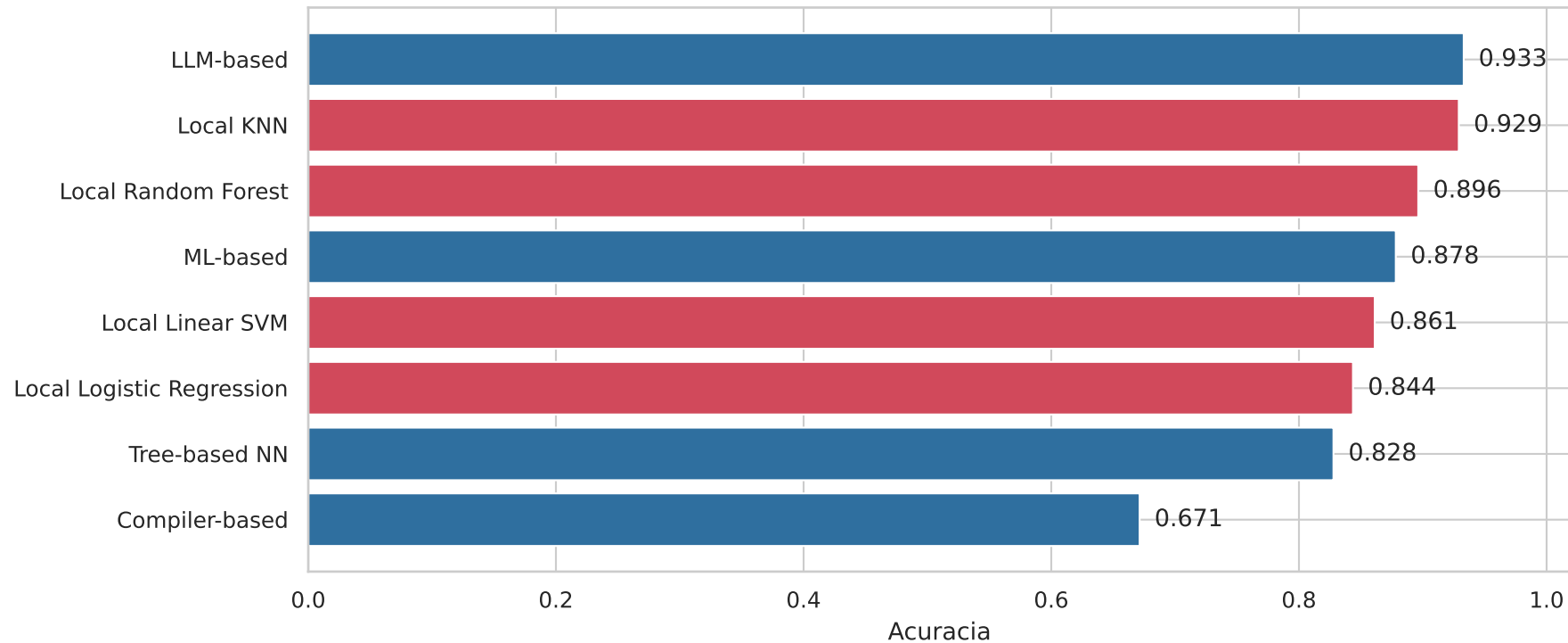
Comparacao: categorias oficiais do artigo e baselines locais reproduzidos
