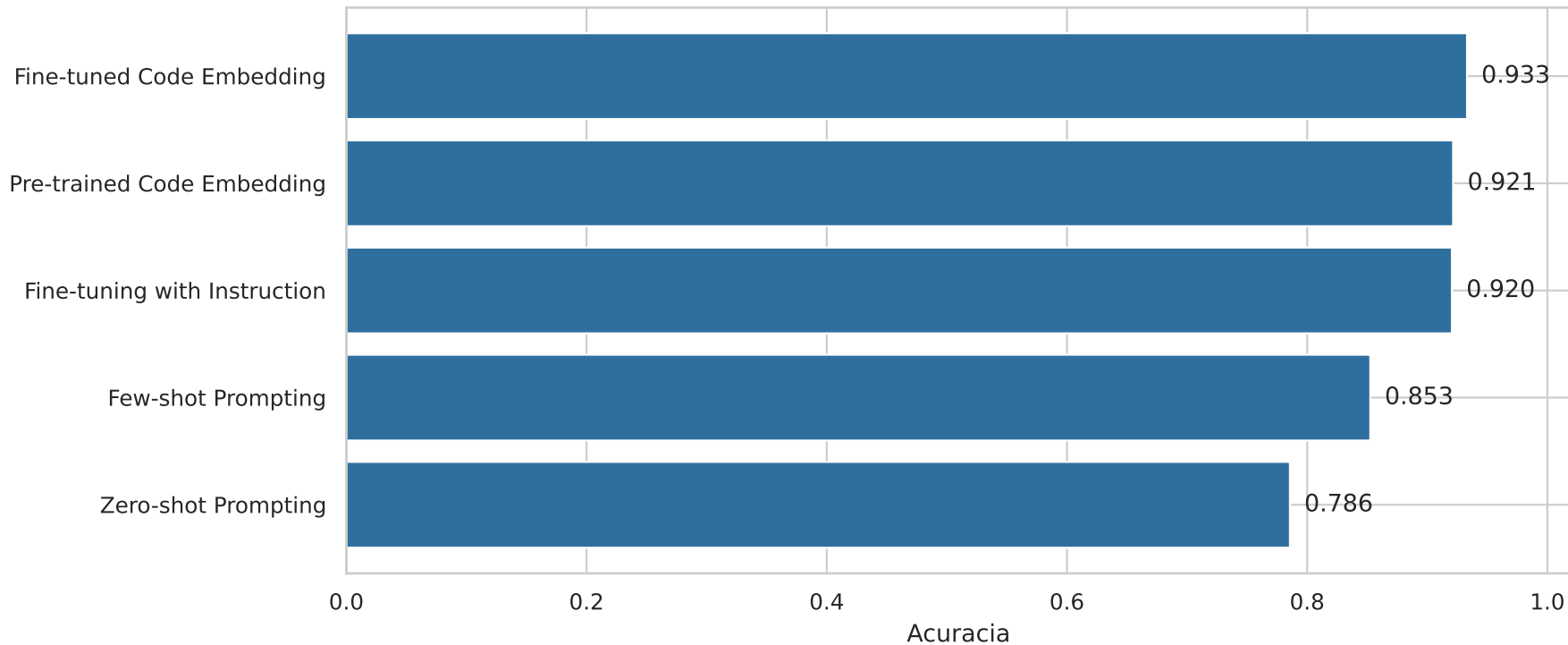
Resultados oficiais por estratégia LLM no pacote do artigo
