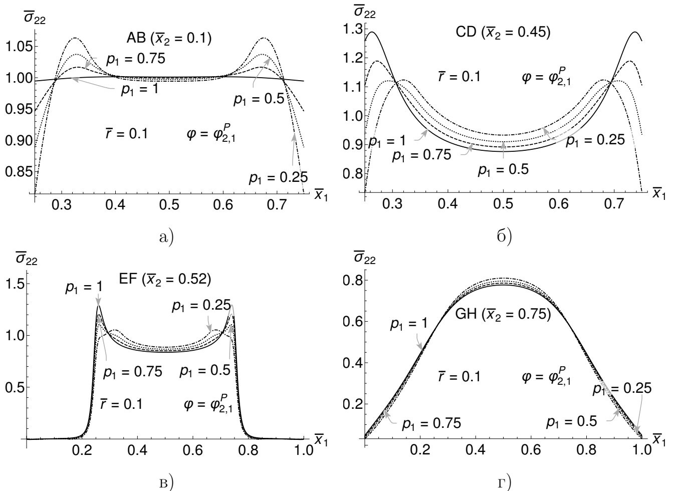
Рис. 4.17. Распределение напряжений \bar{\sigma}_{22} при различных весовых параметрах p_1
