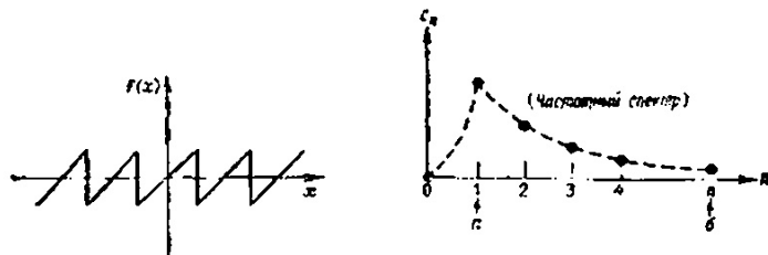
Рис. 11.2. Дискретний частотний спектр пилоподібної функції: а — основна частота (період 2L ), б — n -га гармоніка (період 2L/n ). Послідовність \{c_n\} нагадує спектральний розклад білого світла на кольори. Введемо
