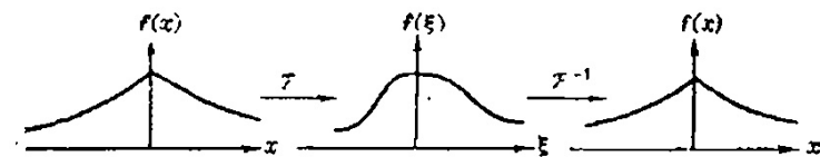
Рис. 12.1. Графіки функції та її образу Фур'є. Наприклад, (див. рис. 12.1)
