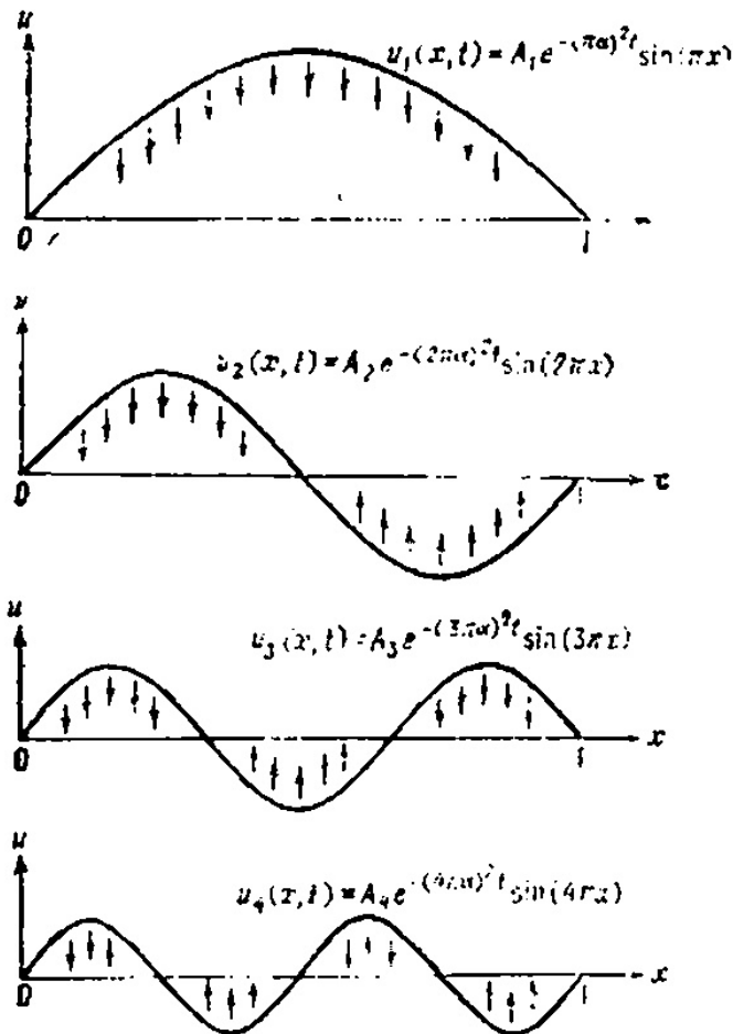
Фіг. 5.3. Фундаментальне рішення u_n(x, t) = A_n e^{-(n\pi\alpha)^2 t} \sin(n\pi x) .
