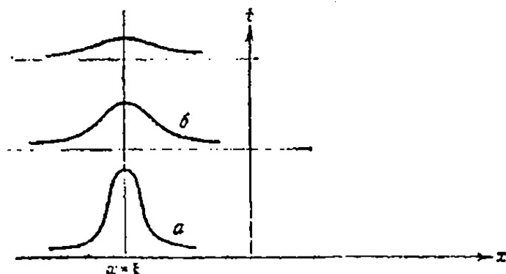
Рис. 12.2. Відгук G(x, t) на тепловий імпульс у точці x = \xi : графік G(x, t) схожий на графік нормального розподілу; зі збільшенням часу максимум зменшується, а крива розширюється. Іншими словами, функція G(x - \xi, t) описує розподіл температури в стрижні в момент часу t , якщо в точці x = \xi подіяв одиничний тепловий імпульс (див. рис. 12.2). Тепер формулі (12.9) можна дати таку інтерпретацію: початкову температуру u(x, 0) = \phi(x) можна подати як неперервну сукупність точкових імпульсів величини \phi(\xi) у точках x = \xi . Кожен точковий імпульс дає розподіл температури \phi(\xi)G(x - \xi, t) . Результируючий розподіл знаходиться підсумовуванням, тобто інтегруванням, температур від точкових джерел за формулою (12.9). Пізніше ми побачимо, що це один із проявів загального принципу суперпозиції.
