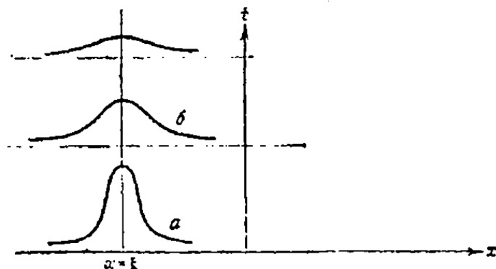
Рис. 12.2. Відгук G(x, t) на температурний імпульс у точці x = \xi . Графік G(x, t) подібний до кривої нормального розподілу; час відіграє роль середньоквадратичного відхилення: при малих t функція вузька, а зі зростанням t помітно розширюється.
