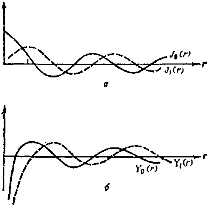
Рис. 30.2 Функції Бесселя. а — функції Бесселя першого рода; б — функції Бесселя второго рода.
