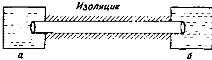
Рис. 3.3. Конвективна теплопередача через межі, а — це рідина при температурі g_1(t) , б — рідина при температурі g_2(t) .
