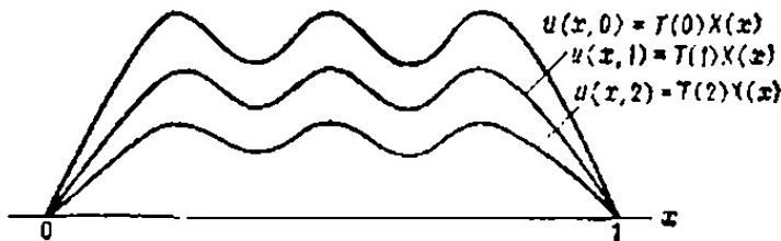
РИСУНОК 5.2 Графік функції X(x)T(t) у різних точках часу t .
