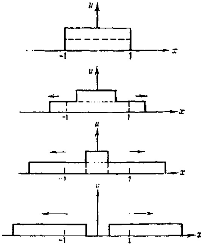
РИС. 17.2. Начальное возмущение распадается на две бегущие волны.
