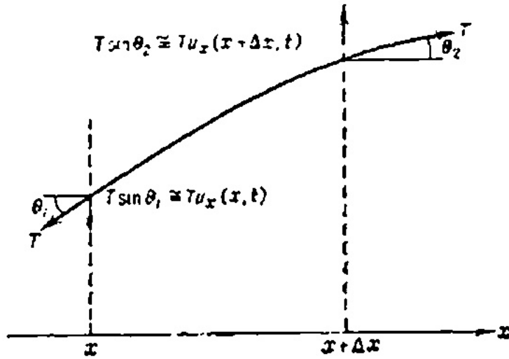
РИС. 16.2. Малый участок (x, x + \Delta x) колеблющейся струны.
