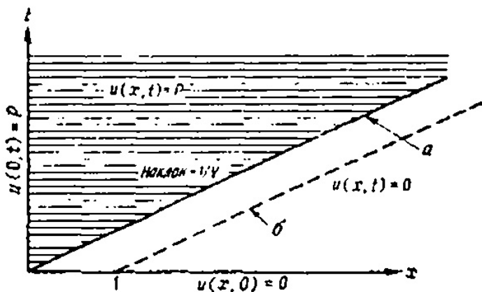
РИС. 15.3 Конвективная волна a — передний фронт примеси, \delta — на одну единицу вперед волнового фронта
