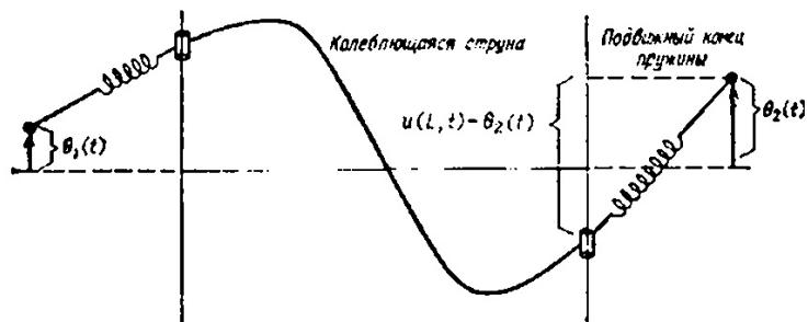
Рис. 19.6. Виникнення неоднорідних граничних умов пружного закріплення: h - коефіцієнт жорсткості пружини. Для умов пружного закріплення однорідні граничні умови часто записують у вигляді
