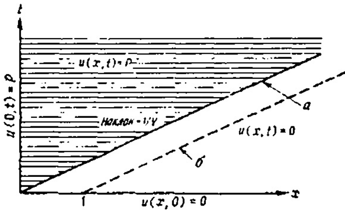
Фіг. 15.3 Конвективна хвиля а — попереду фронту домішок δ — одна одиниця попереду фронту хвиль
