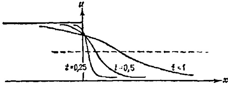
РИС. 15.7. Решение задачи конвективной диффузии. Вещество одновременно движется и диффундирует. (На рис. 15.7 показано, как расплывается передний фронт концентрации.)
