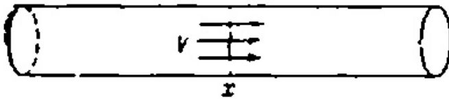
Рис. 15.1. Количество вещества, переносимого в одну секунду через поперечное сечение в точке x за счет конвекции, равно Vu(x, t) .
