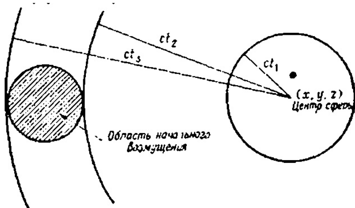
24.3. Схема поясняет, как начальное возмущение влияет на точку (x, y, z) .
