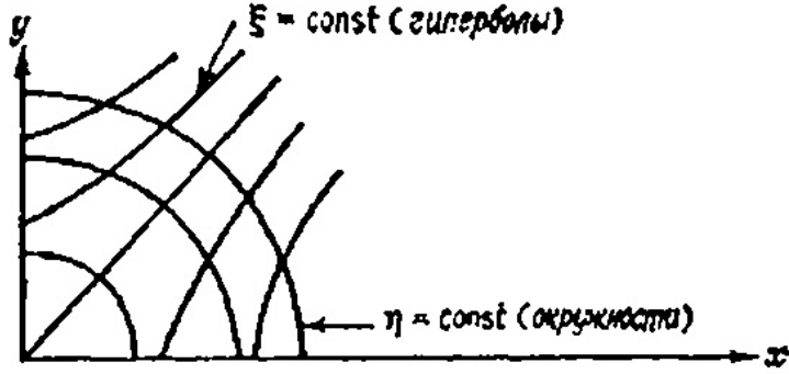
Фіг. 23.3. Нові координати карактора.
