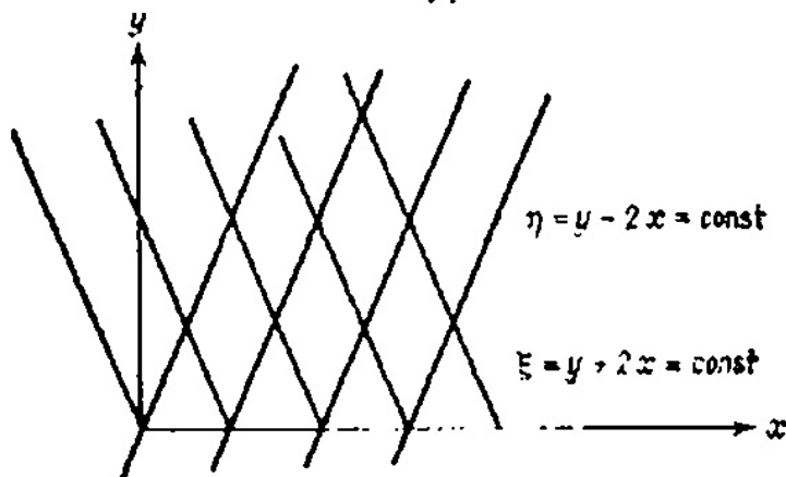
Фіг. 23.2. Характеристичні координати рівняння u_{xx} - 4u_{yy} + u_x = 0 .
