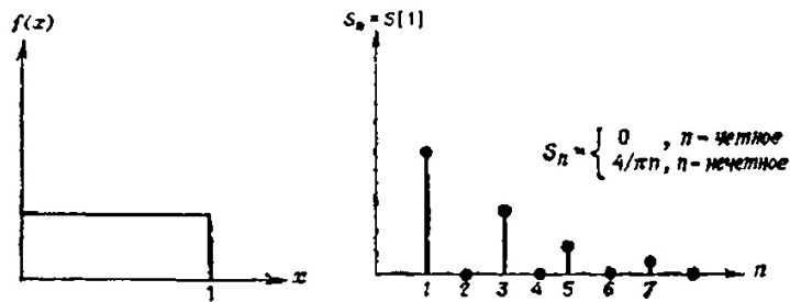
с. 25.1. Графики функции f(x) = 1 и ее преобразования.
