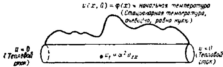
Фіг. 5.1. Схематичне представлення проблеми дифузії.
