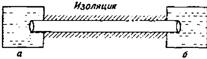
Фіг. 3.3. Конвективний теплообмін через межу, а — джерело рідини при температурі g_1(t) , б — радін при температурі g_2(t) .
