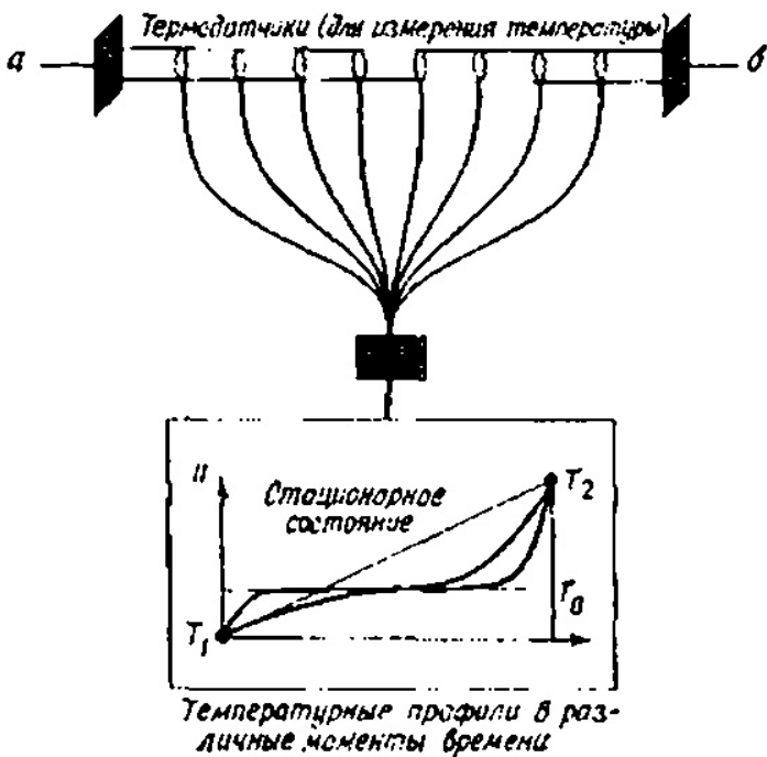
Фіг. 2.1. Схема експерименту: а – температура термопар, яка є температурою T_1 на лівому вітрі стрижка; б — це ціна термопар, тобто температура T_2 на правій лаві стрижка.
