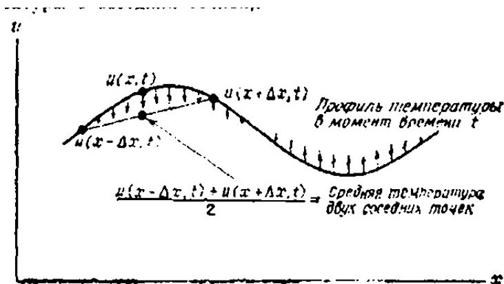
Фіг. 2.2. Стрілки показують зміну температури від часу до рівня u_t = \alpha^2 u_{xx} .
