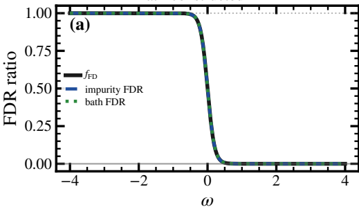
Nonthermal eigenmode diagnostic
