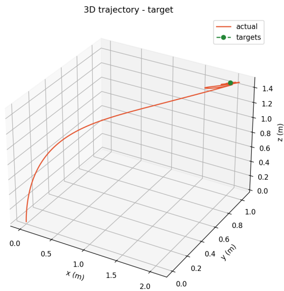
图 1 单目标点实验的三维实际轨迹与目标
