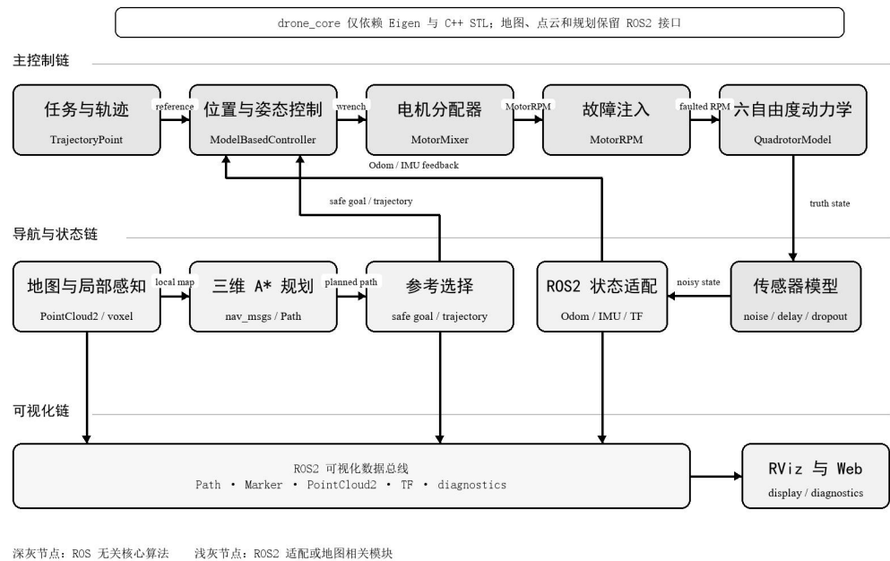
图 1 系统节点与主要数据流
