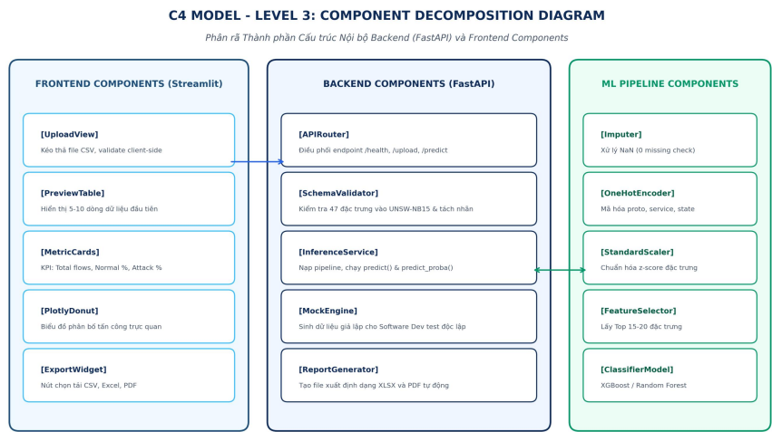
Figure 3: Sơ đồ Phân rã Thành phần Nội bộ (C4 Model - Level 3: Component Decomposition Diagram)
