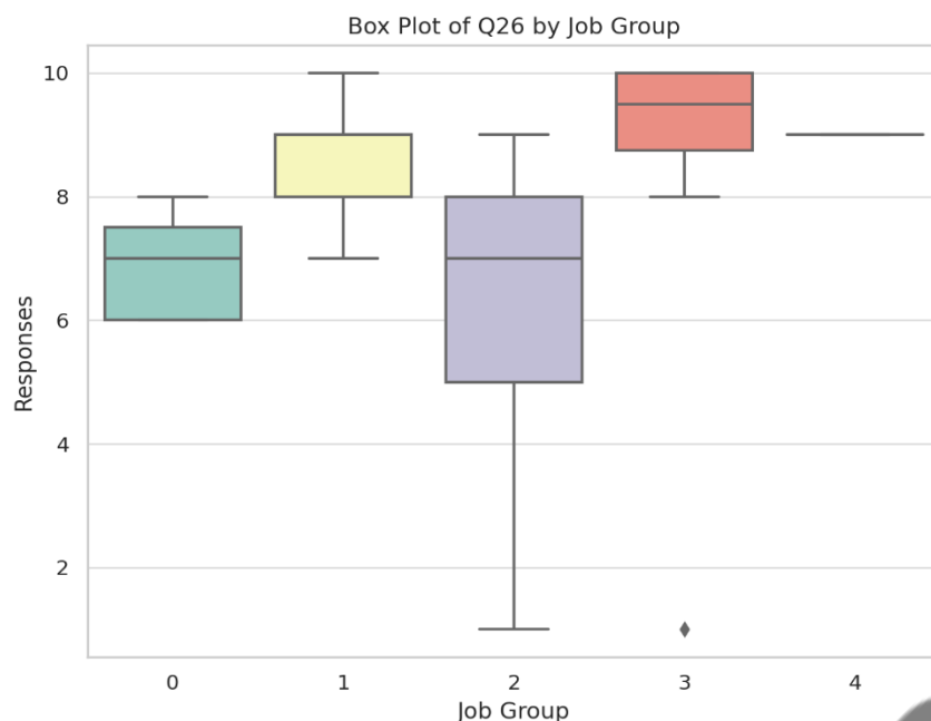
Figure 27 : Box-plot par groupe Q26
