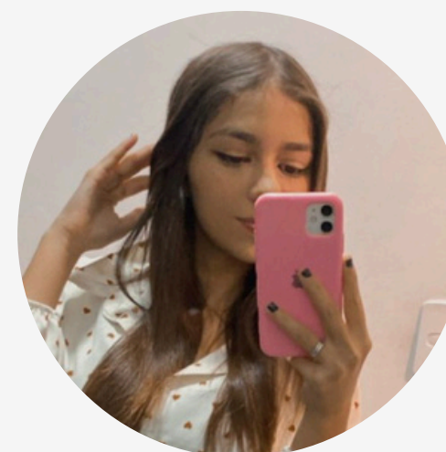
Thais Pereira
