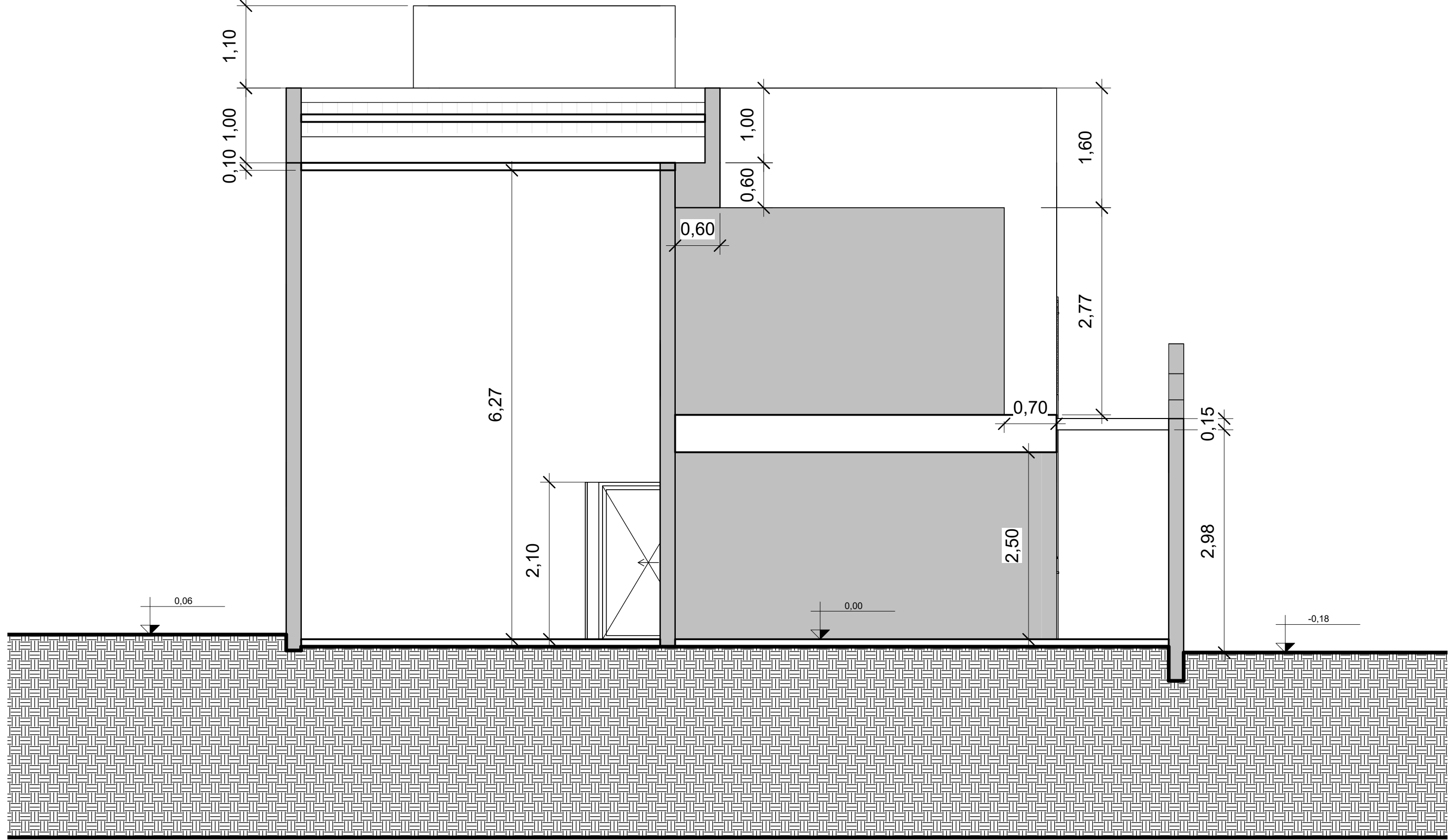
2 CORTE AA 1:50
