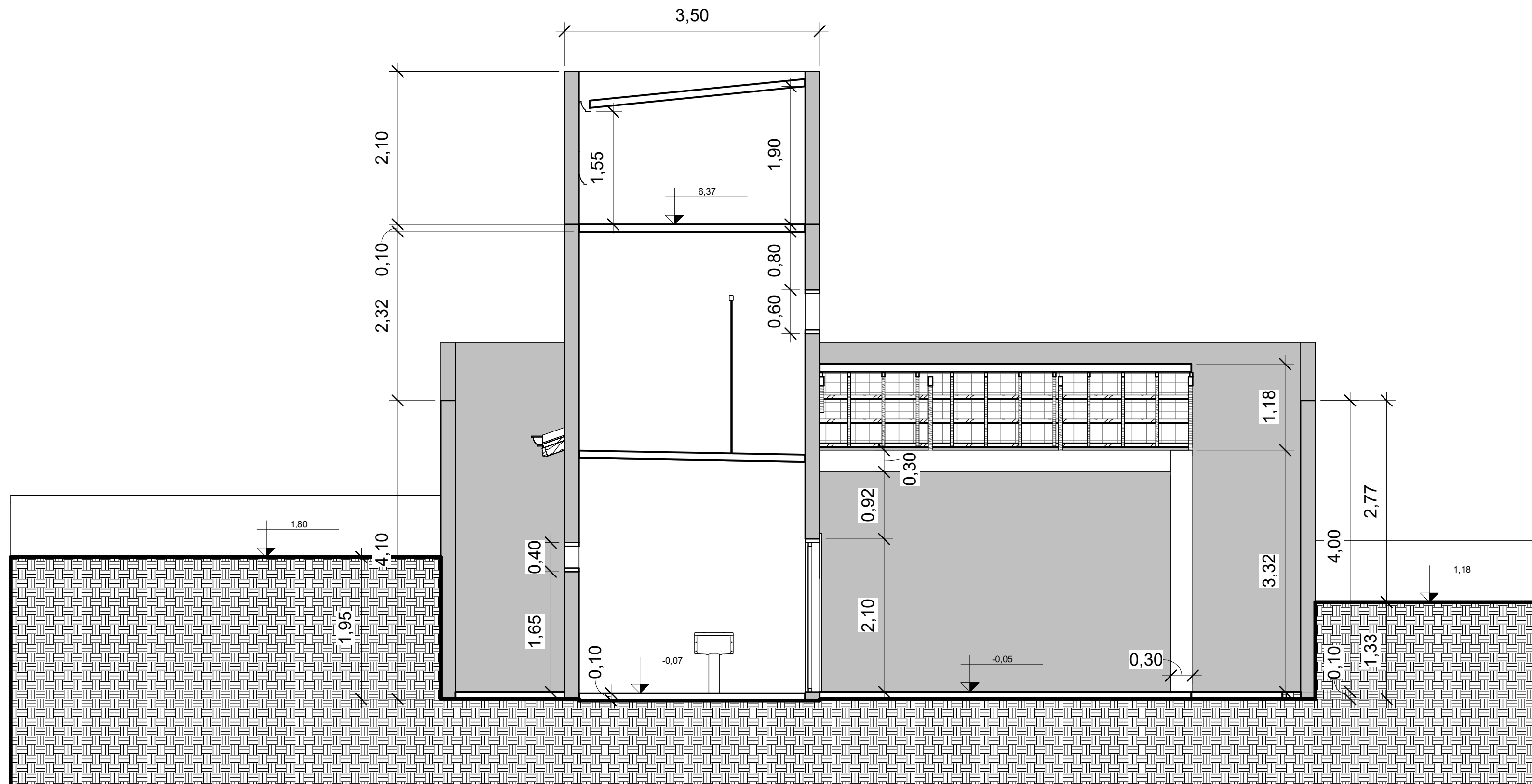
4 CORTE CC 1:50
