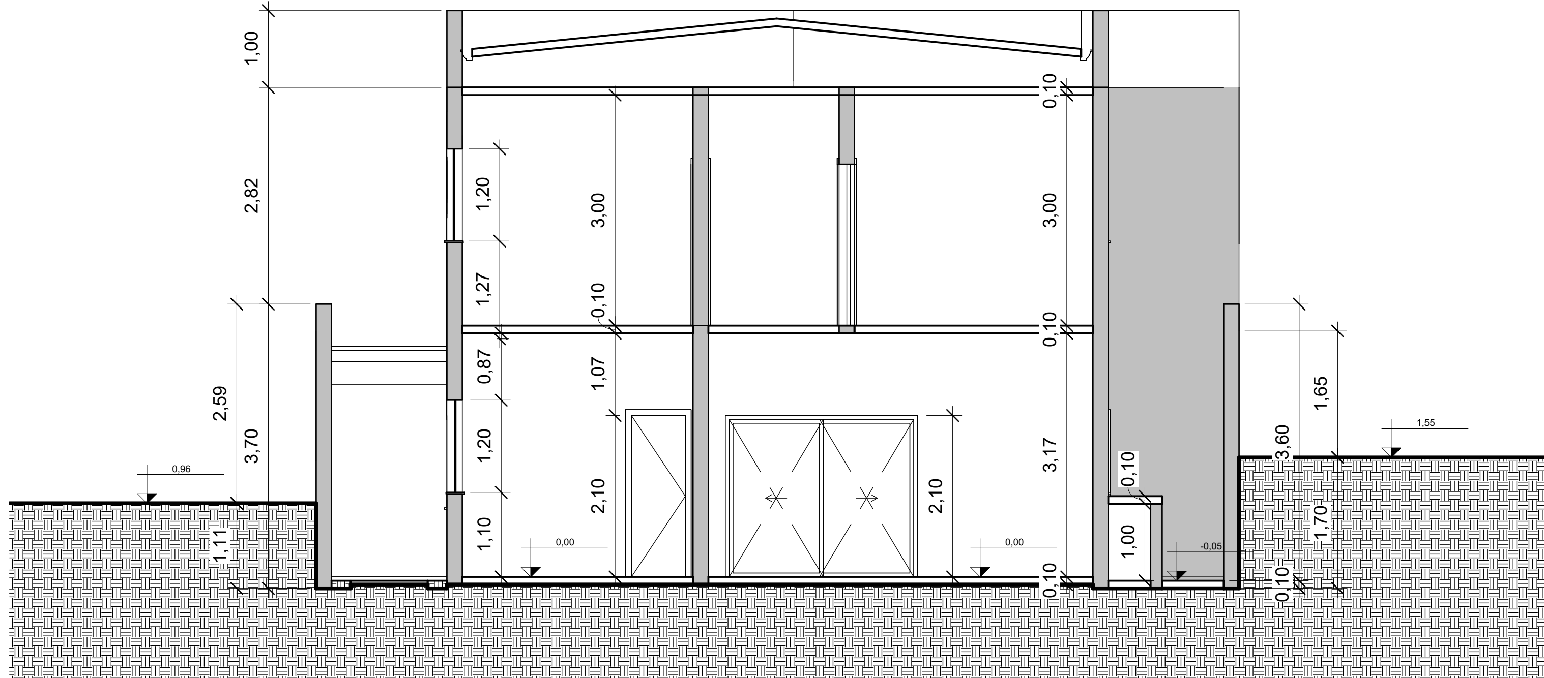
3 CORTE BB 1:50
