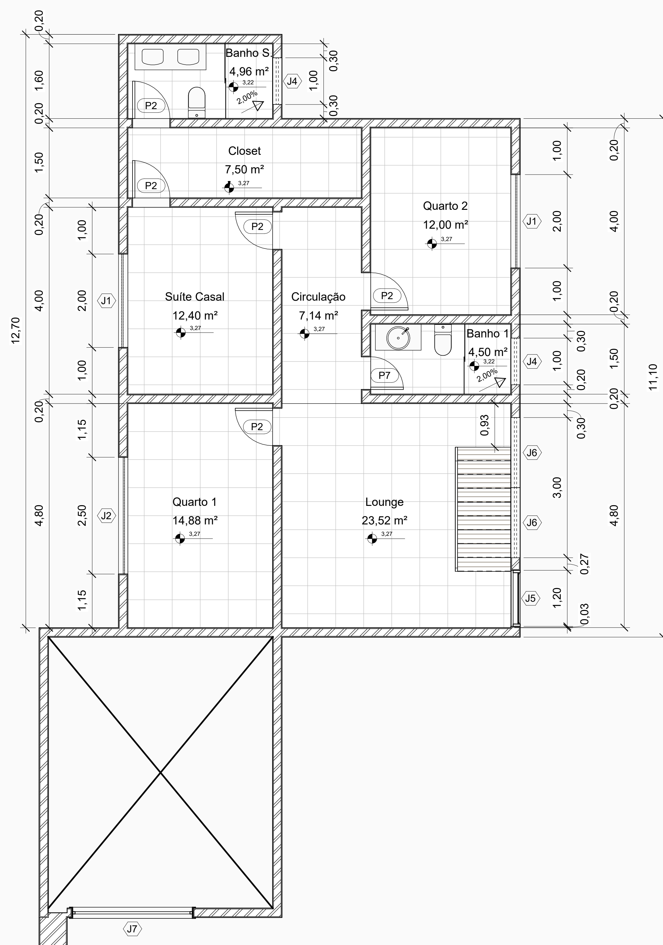
4 PLANTA BAIXA PAV. SUPERIOR 1 : 50
