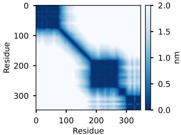
O75764 \sigma(r) Sim.
