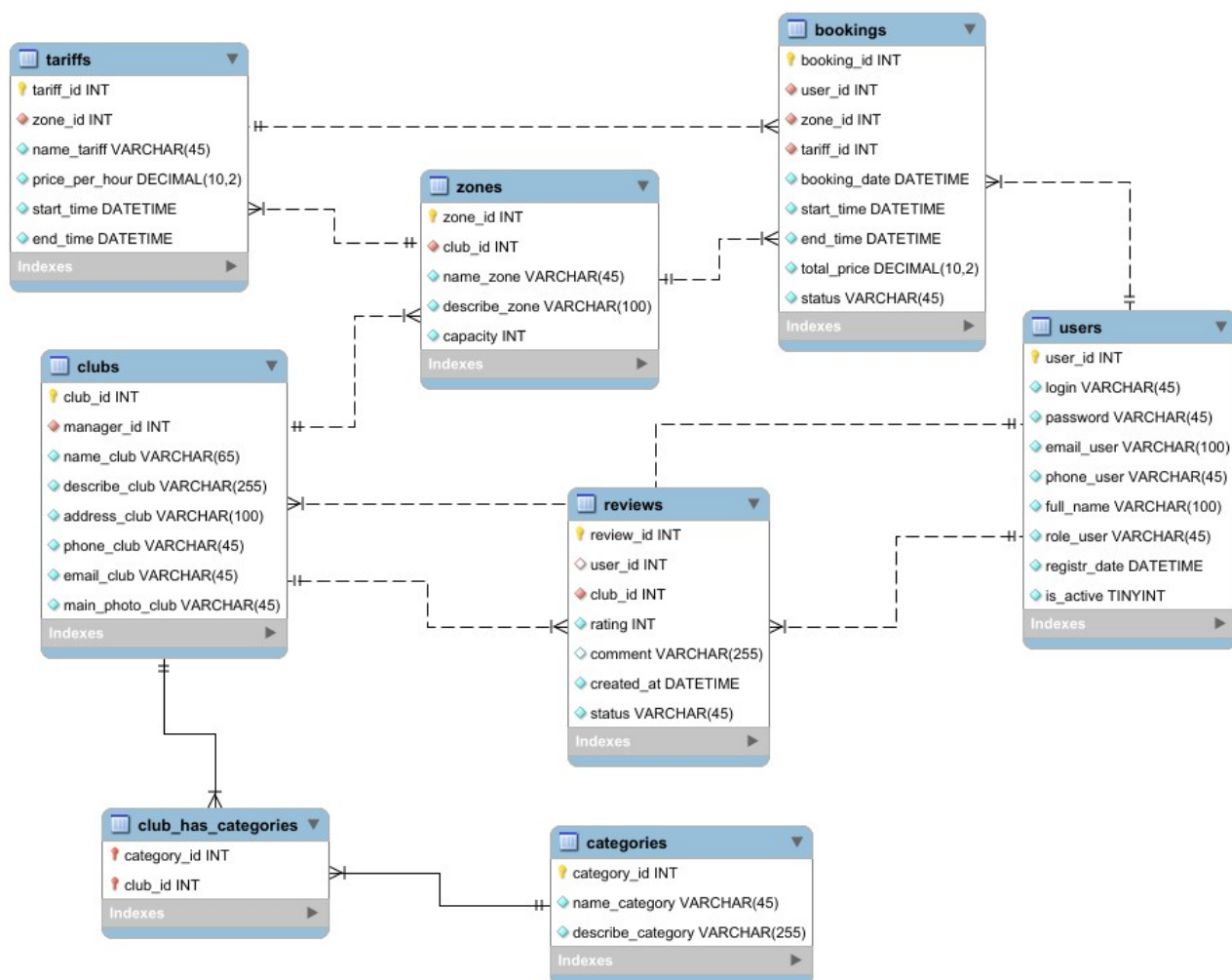
Рисунок 1.6.8 – ER-диаграмма
