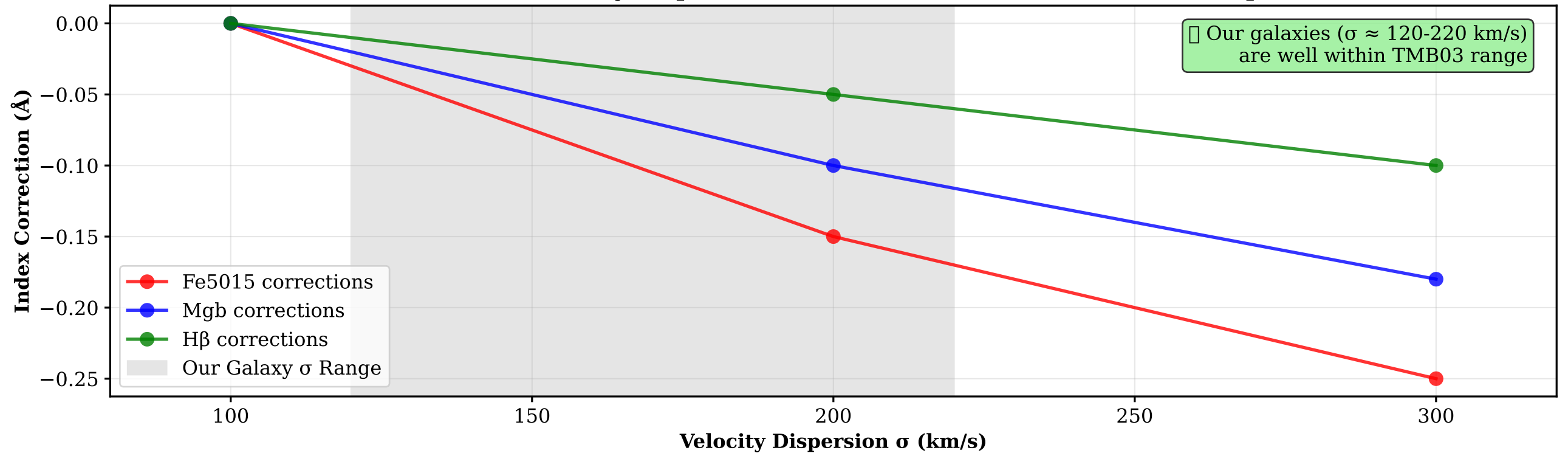
(d) TMB03 Velocity Dispersion Corrections - Validation for Our Sample
