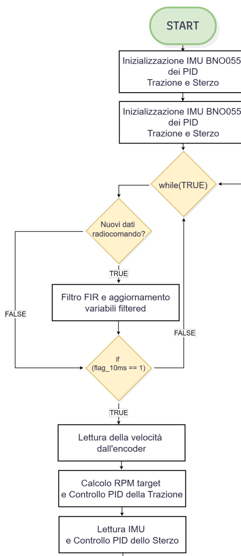
Figure 4.1: Diagramma di flusso del codice sviluppato
