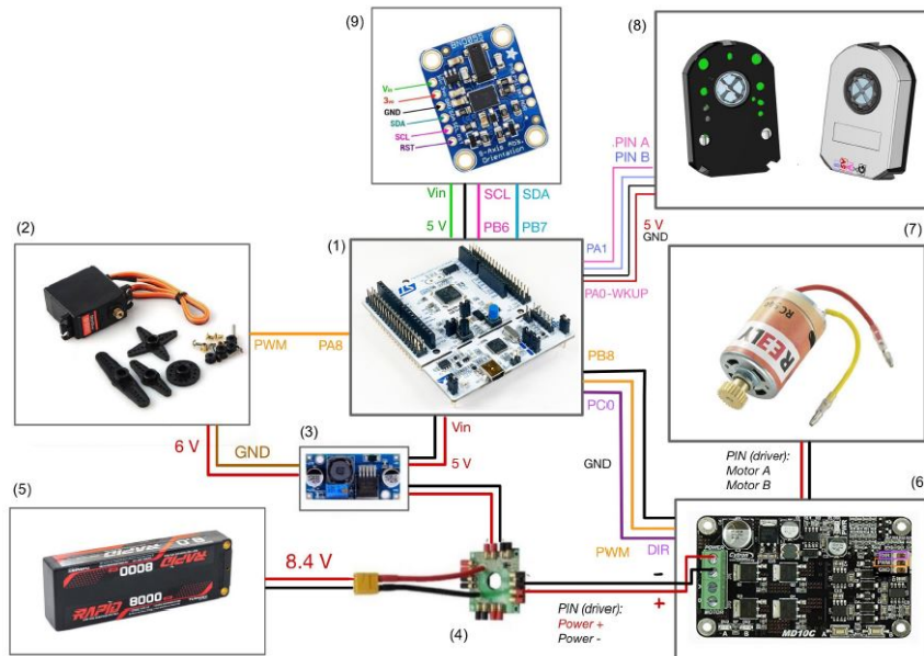
Figure 2.12: Schema dei collegamenti
