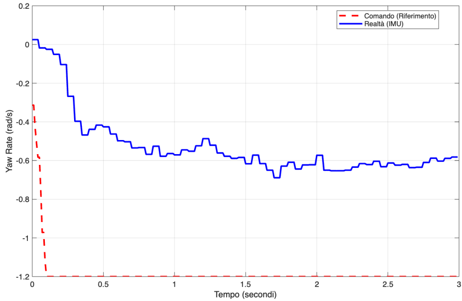
Figure 5.16: Risposta a gradino del controllo di sterzo, riferimento di -1.2 rad/s.
