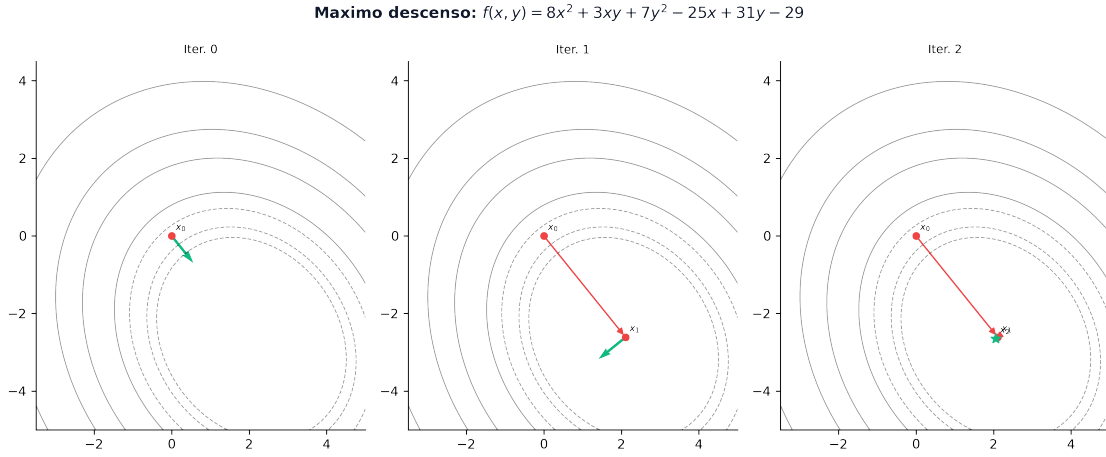
Figura 2.13: Máximo descenso: secuencia de iteraciones mostrando trayectoria ortogonal sobre las curvas de nivel elípticas
