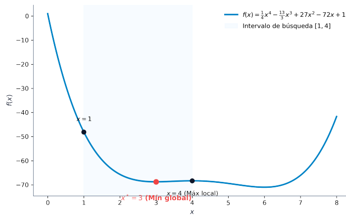
Figura 2.3: Caso de prueba para métodos de búsqueda 1D: función de cuarto grado y su mínimo global
