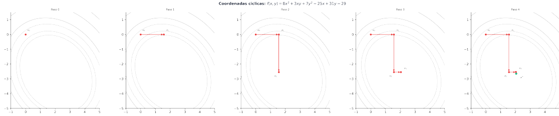
Figura 2.12: Trayectoria en escalera del descenso por coordenadas cíclicas sobre una función cuadrática acoplada
