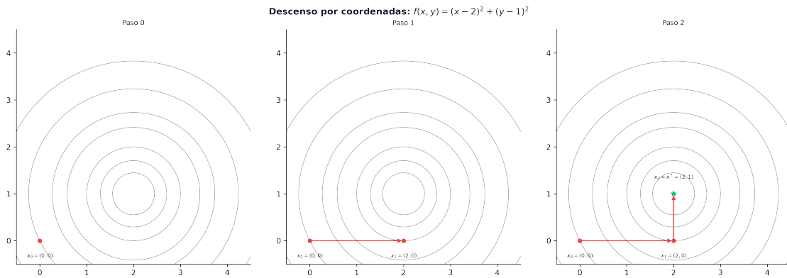
Figura 2.11: Descenso por coordenadas cíclicas: secuencia de pasos sobre curvas de nivel circulares
