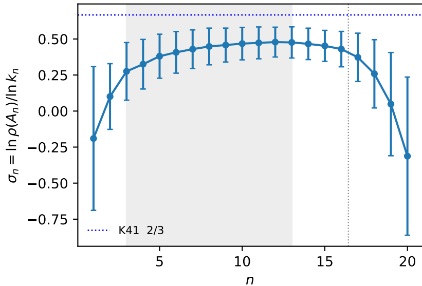
(b) pole abscissa per shell (mean \pm sd)
