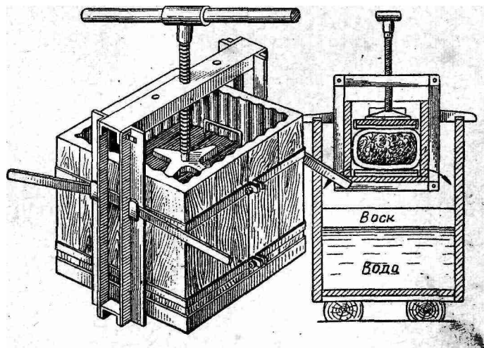
Рис. 70. Деревянный воскопресс конструкции В. А. Темнова.
