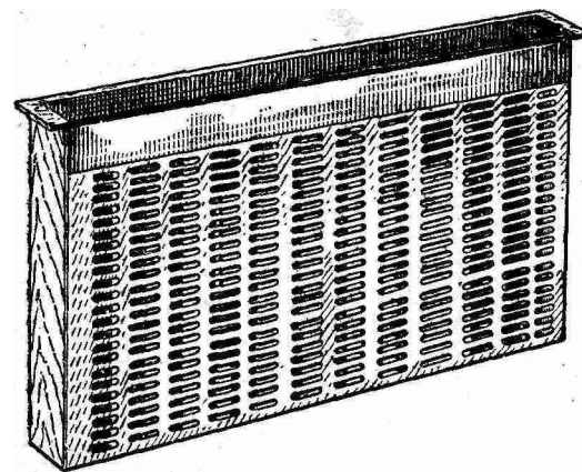
Рис. 84. Однорамочный изолятор из разделительной решетки для получения одновозрастного расплода.
