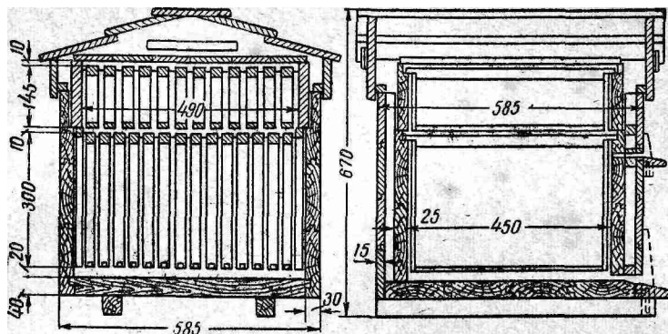
Рис. 46. Устройство утепленного 14-рамочного улья.
