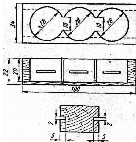
Рис. 89. Клеточка для почтовой пересылки маток:
