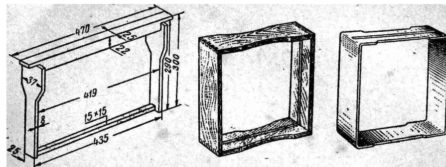
Рис. 37. Гнездовая рамка.
