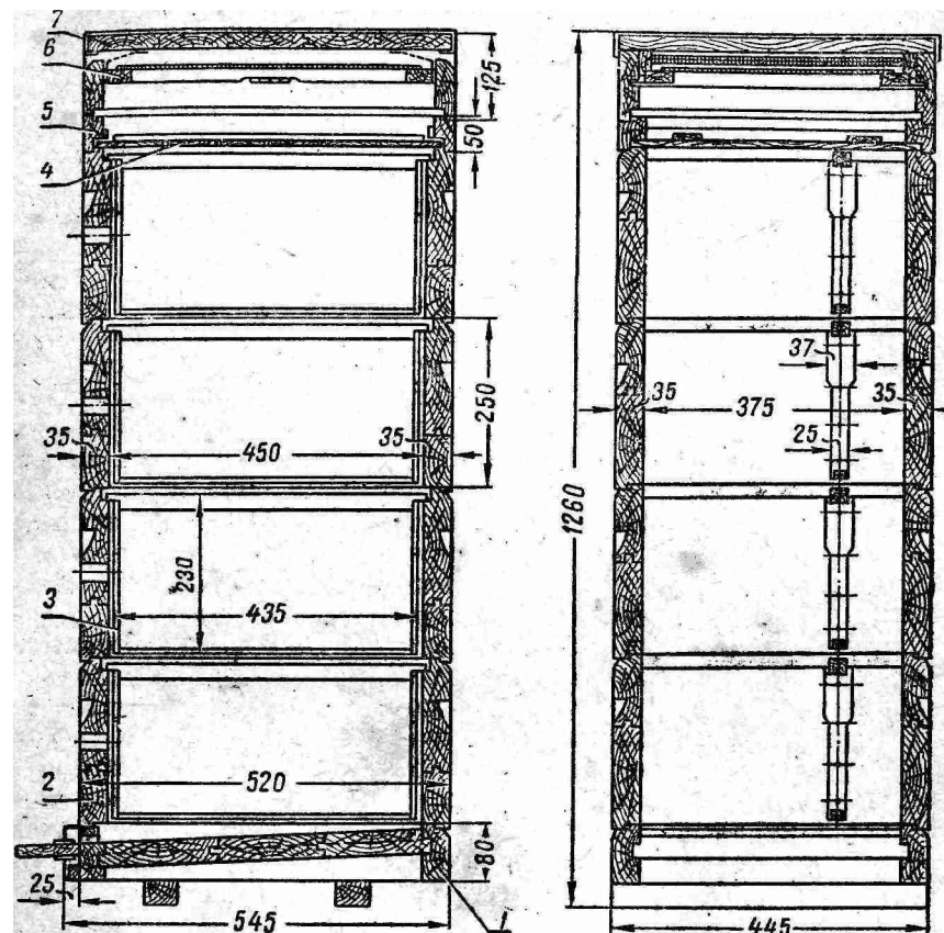
Рис. 41. Устройство многокорпусного улья:
