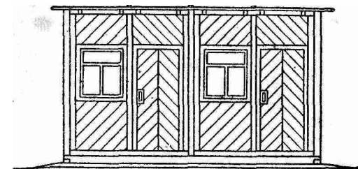
Рис. 34. Разборный домик для кочевых пасек.
