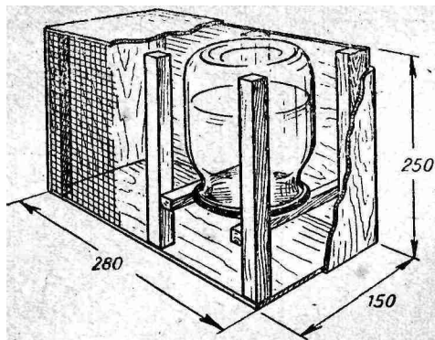
Рис. 93. Бессотовый пакет для транспортировки пчел (размеры в мм).
