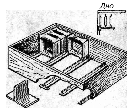
Рис. 39. Магазин с пластинками в форме перевернутой буквы Т.
