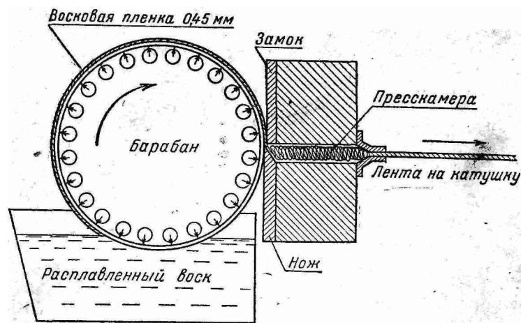
Рис. 114. Схема работы лентообразующей машины.
