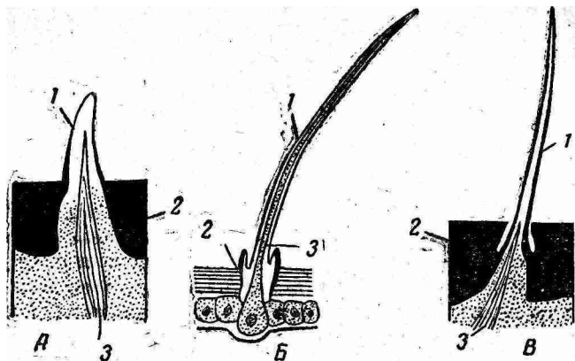
Рис. 10. Органы осязания пчелы:
