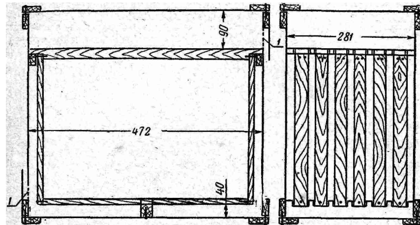
Рис. 92. Продольный и поперечный разрез пакета для дальней транспортировки пчел (1 — темная вентиляция; размеры в мм).
