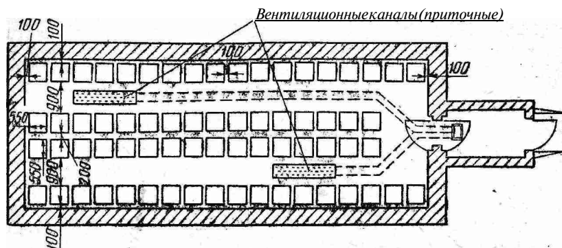
Рис. 26. Схема размещения ульев в зимовнике (размеры в мм).
