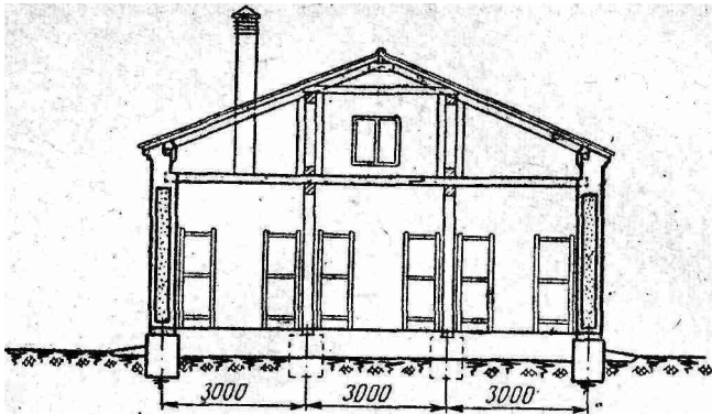
Рис. 31. Поперечный разрез надземного зимовника на 300 пчелиных семей (стены кирпичные колодцевой кладки; размеры в мм).
