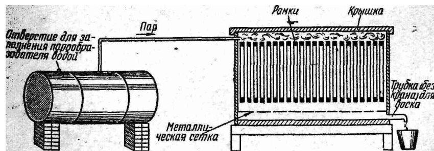
Рис. 72. Схема паровой пасечной воскотопки.
