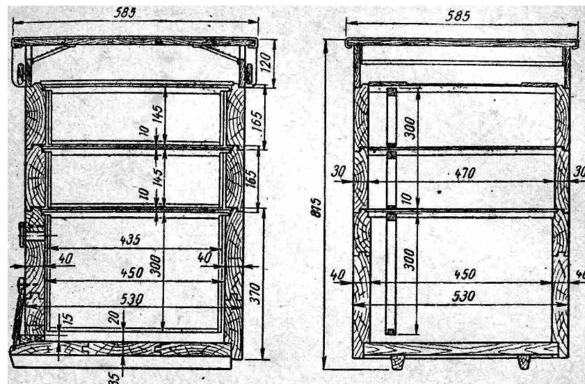
Рис. 43. Устройство однокорпусного улья с двумя магазинами: с л е в а — разрез вдоль рамок; с п р а в а — разрез поперек рамок.
