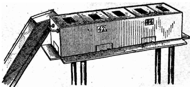
Рис. 88. Маломерный пятиместный нуклеус.
