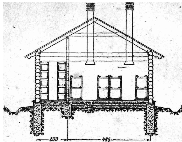
Рис. 28. Поперечный разрез надземного зимовника на 162 пчелиные семьи с сотохранилищем (размеры в см).
