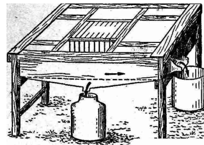
Рис. 63. Стол для распечатывания сотов, предложенный В. А. Темновым.
