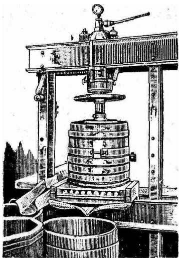
Рис. 113. Гидравлический пресс на воскоперерабатывающем заводе.
