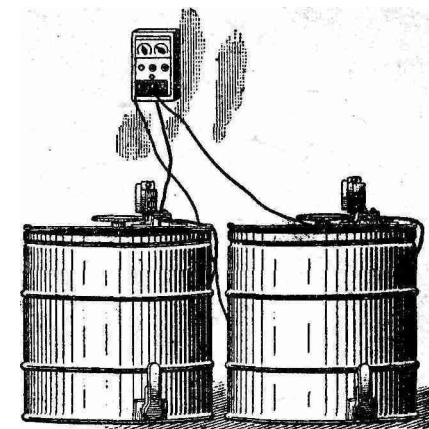
Рис. 66. Спаренные медогонки с электроприводом.
