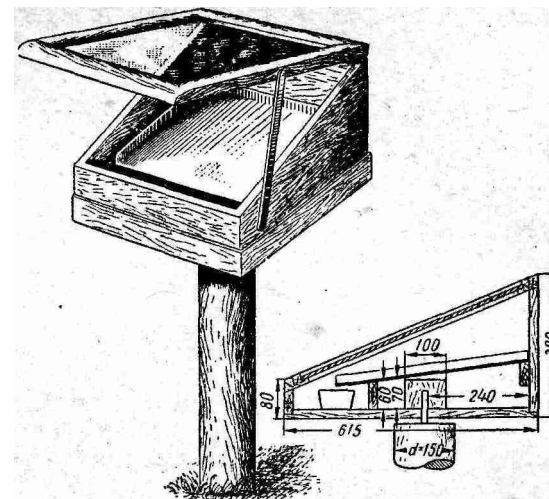
Рис. 71. Солнечная воскотопка.
