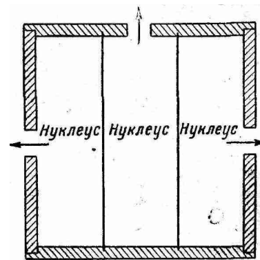
Рис. 87. Схема трехместного нуклеусного улья.
