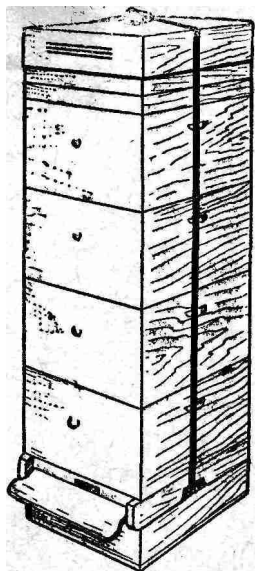
Рис. 94. Многокорпусный улей, стянутый ленточным скрепом с катушечным замком.
