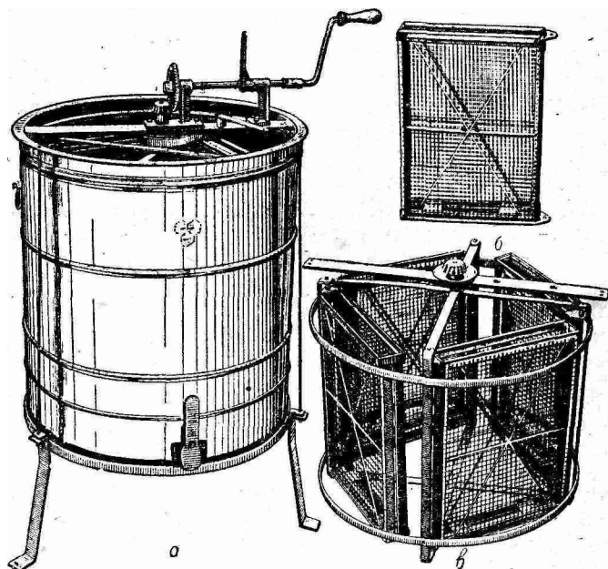
Рис. 64. Хордиальная четырехрамочная оборотная медогонка: а — общий вид; б — кассета; в — ротор с кассетами.
