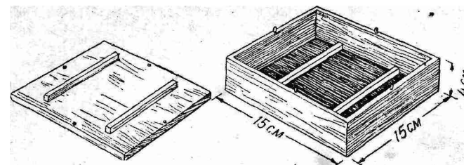
Рис. 112. Ящик для пересылки сота с пораженным расплодом.
