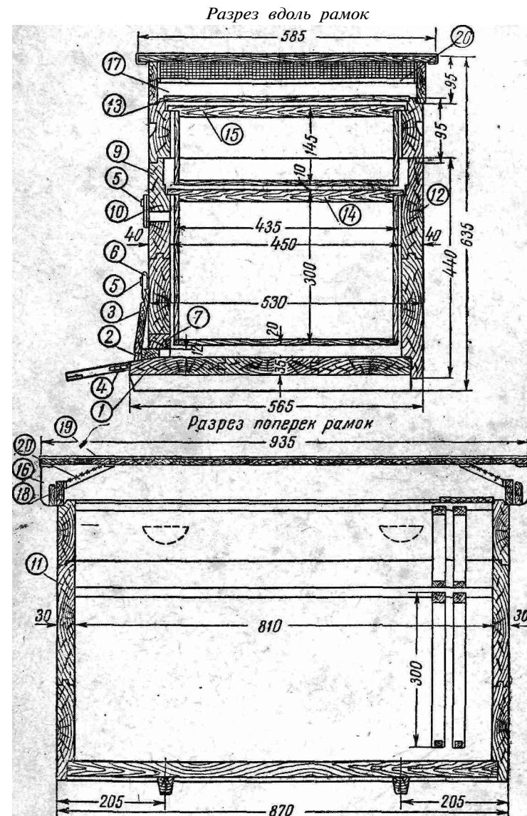
Рис. 45. Устройство лежака на 20 рамок:
