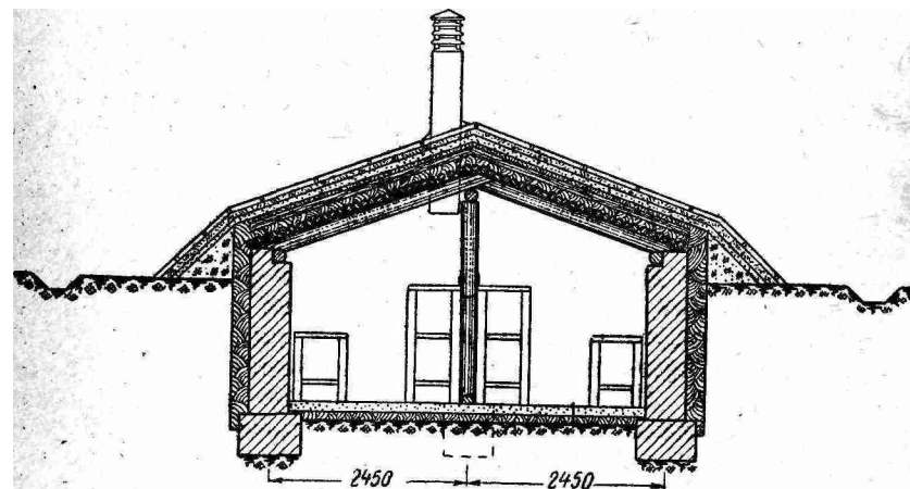
Рис. 27. Поперечный разрез подземного зимовника на 108 пчелиных семей (размеры в мм).
