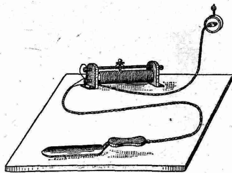
Рис. 61. Электрический нож, включенный в сеть через реостат.
